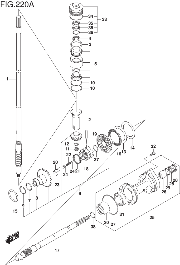
FIG. 220A (1-D-11) トランスミッション
