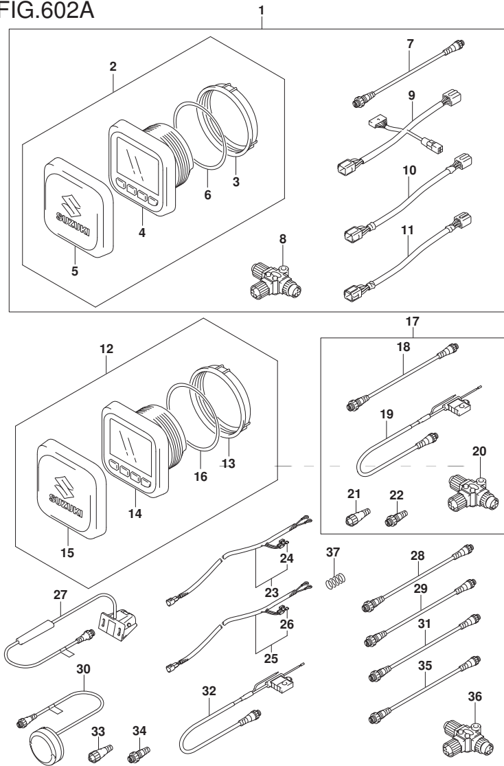
FIG. 602A (1-H-8) オプション:マルチ ファンクション ゲージ (2)
