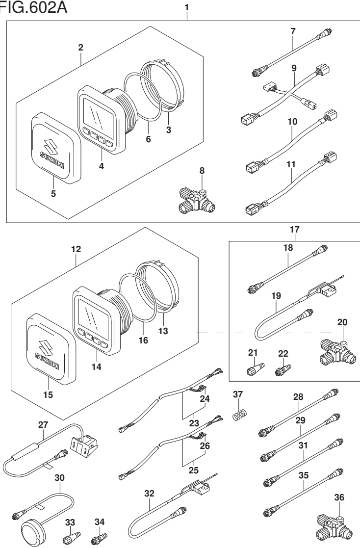
FIG. 602A (1-H-9) オプション:マルチ ファンクション ゲージ (2)
