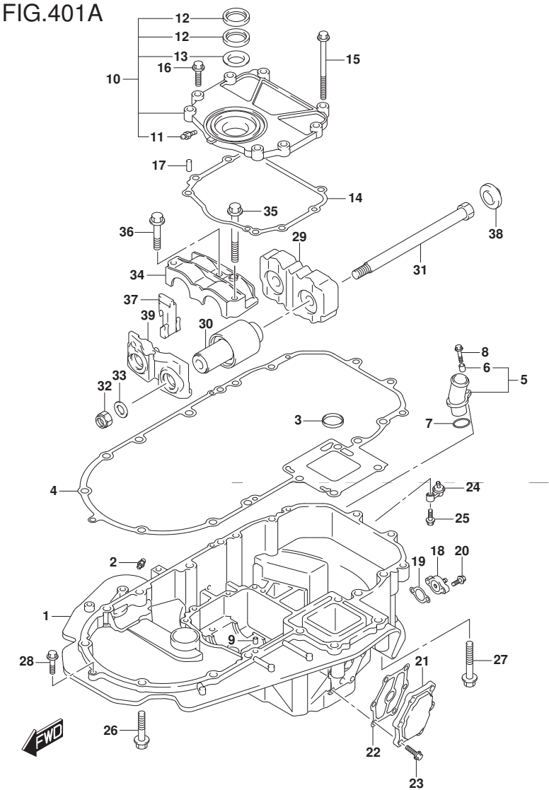
FIG. 401A (1-F-4) エンジンホルダー
