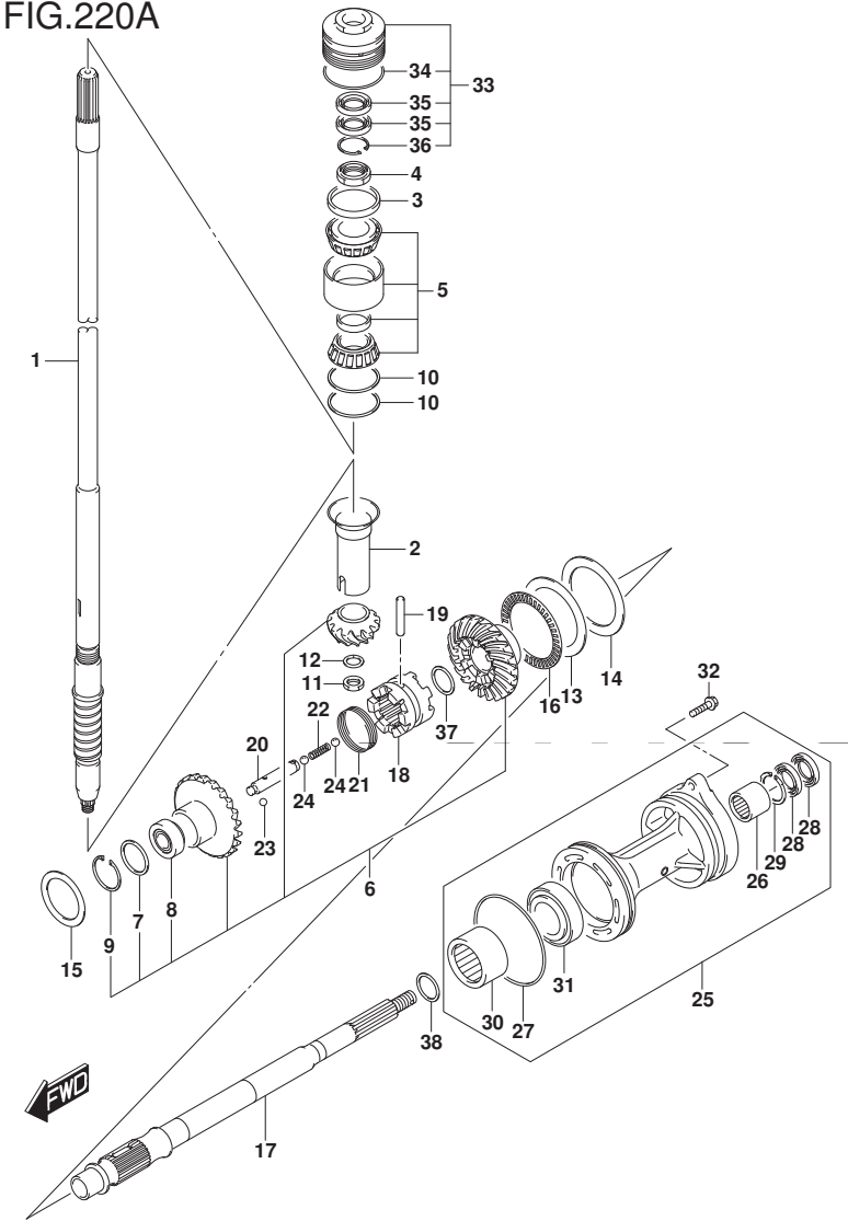
FIG. 220A (1-D-8) トランスミツシヨ
