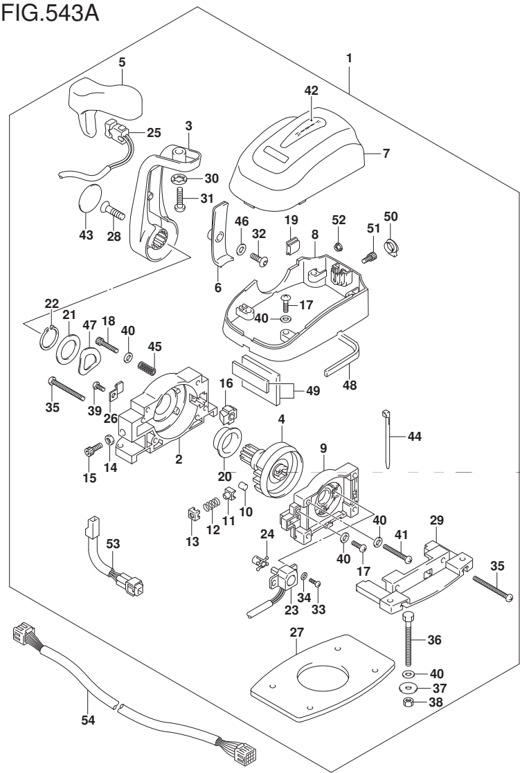
FIG. 543A (1-H-4) オプション:リモート コントロール アッシ シングル
