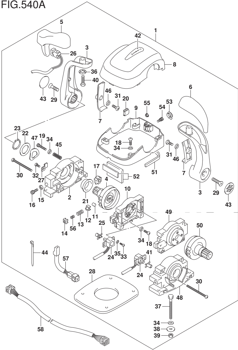
FIG. 540A (1-G-14) オプション:リモート コントロール アツシ デュアル
