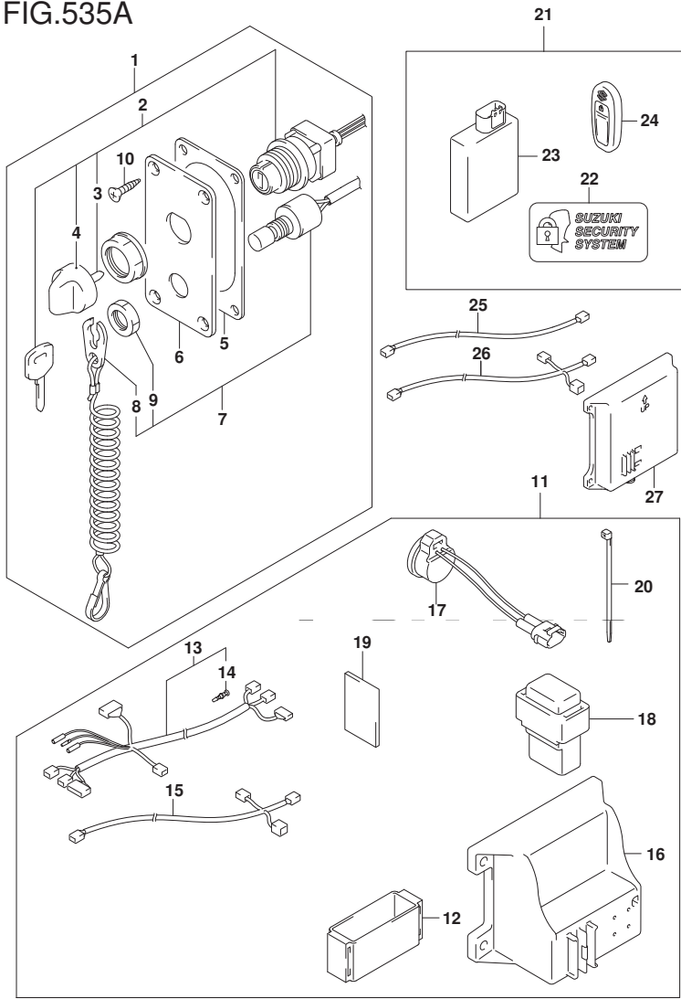
FIG. 535A (1-G-13) オプション:キーレススタート
