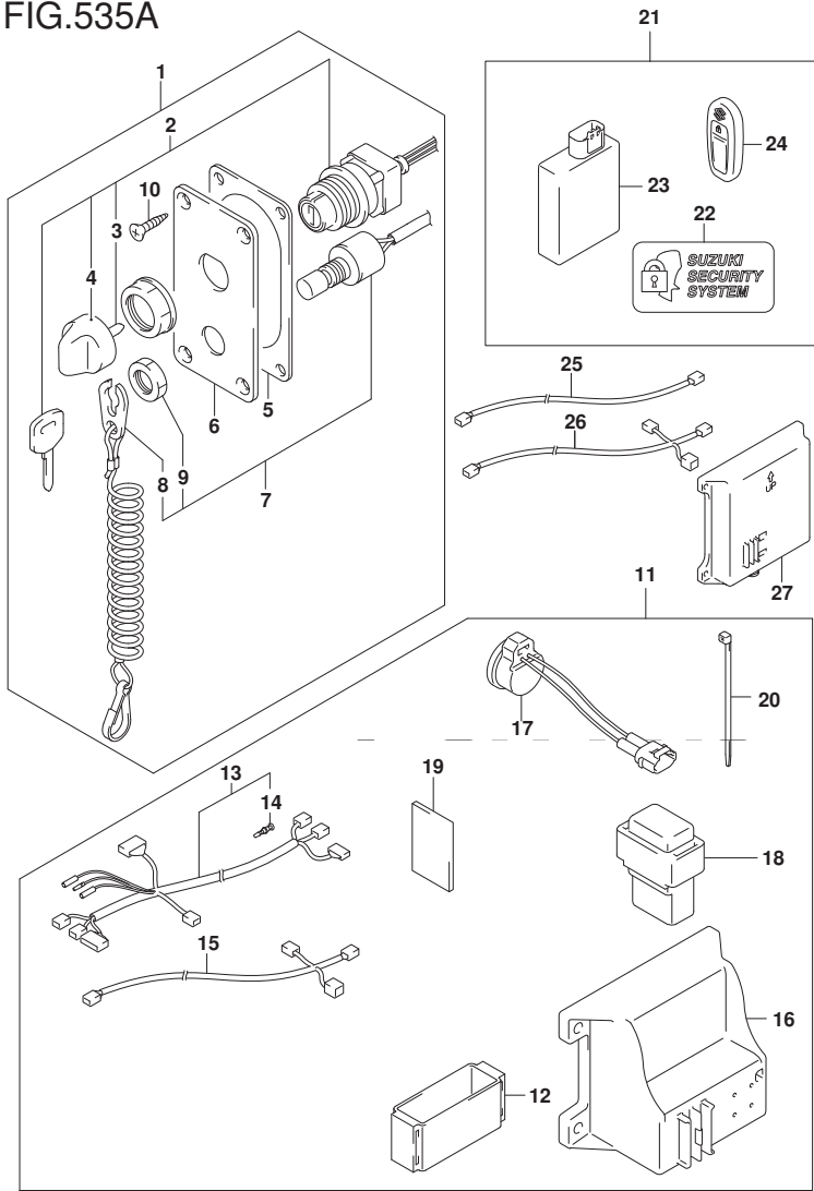
FIG. 535A (1-G-12) オプション:キーレススタート
