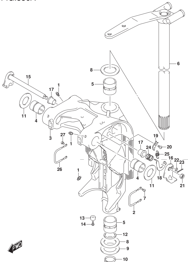
FIG. 336A (1-E-12) スイベル ブラケット
