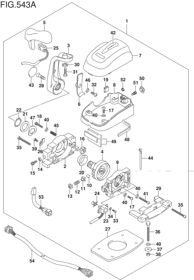
FIG. 543A (1-H-3) オプション:リモート コントロール アツシ シングル
