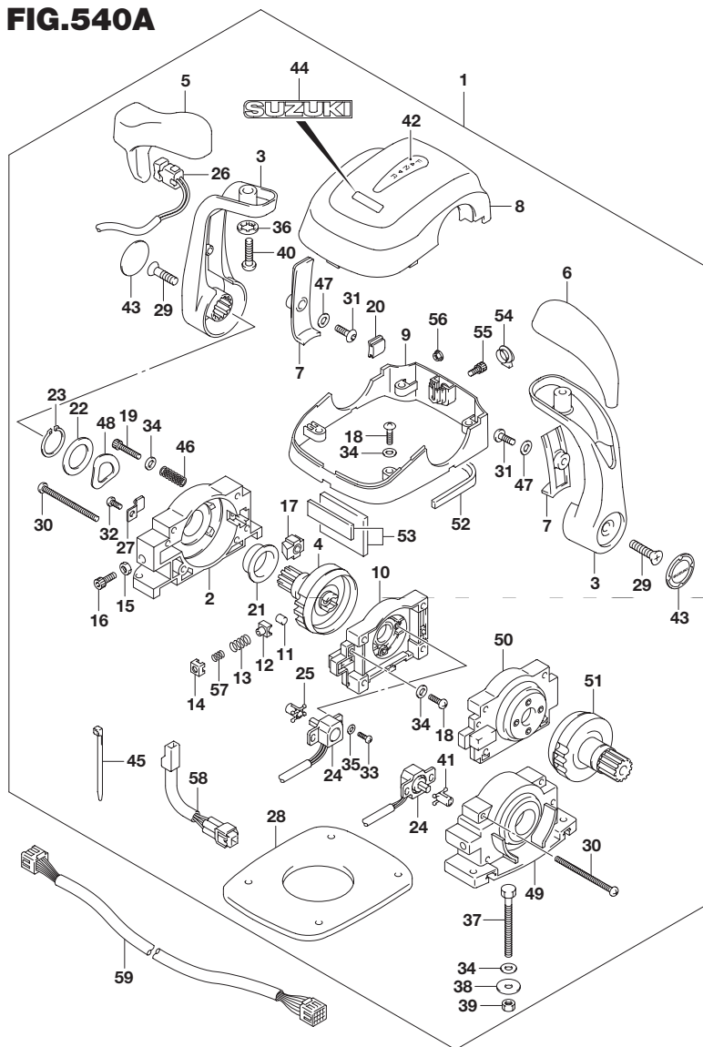
FIG.540A (1-F-15) オプション:リモートコントロール アッシ デュアル
