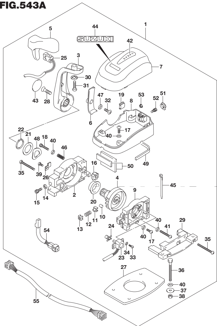
FIG.543A (1-G-2) オプション:リモートコントロール アッシ シングル
