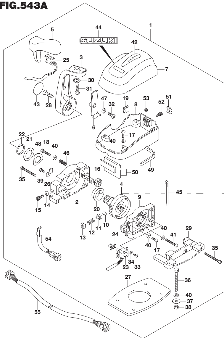
FIG.543A (1-G-4) オプション:リモートコントロール アッシ シングル
