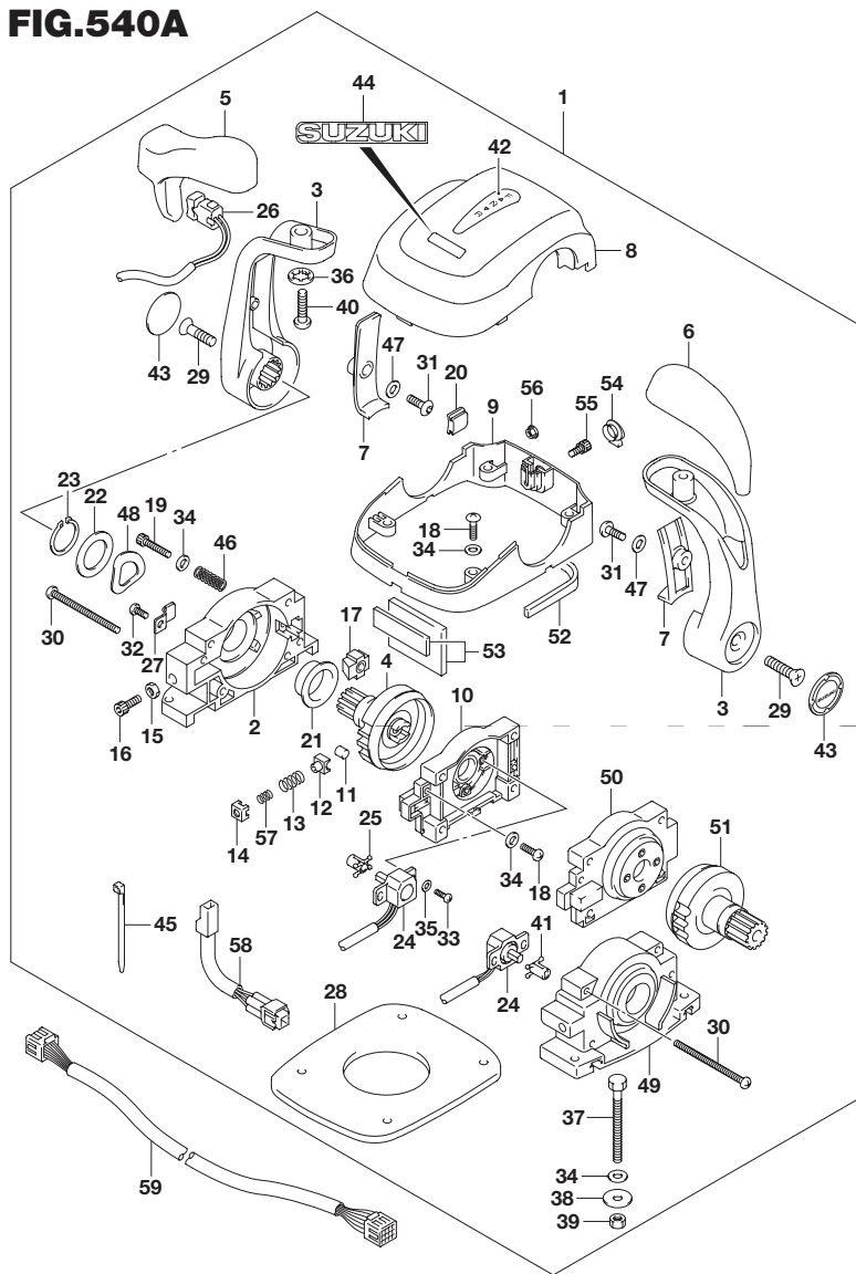
FIG.540A (1-F-14) オプション:リモートコントロール アッシ デュアル
