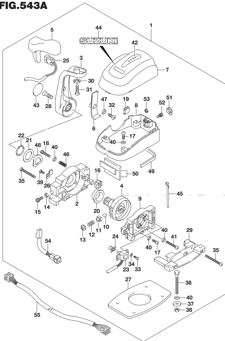
FIG.543A (1-G-3) オプション:リモートコントロール アッシ シングル
