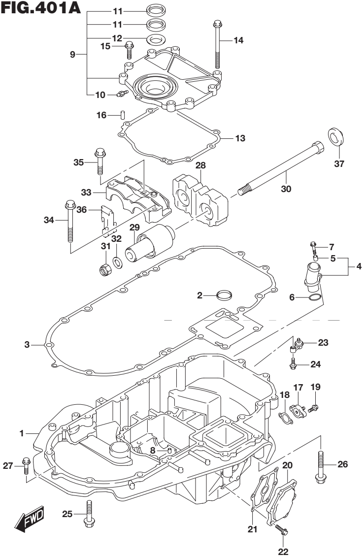
FIG.401A (1-E-7) エンジン ホルダ
