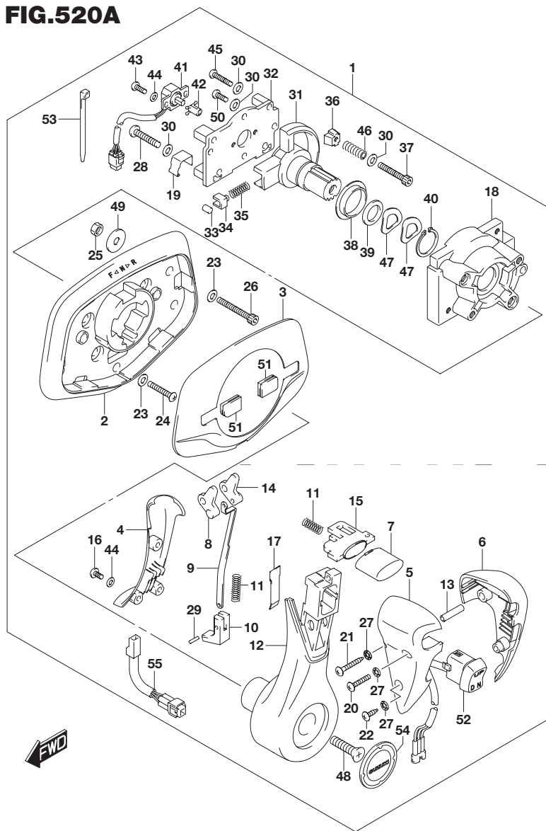
FIG.520A (1-F-5) オプション:フラッシュ マウントリモコン
