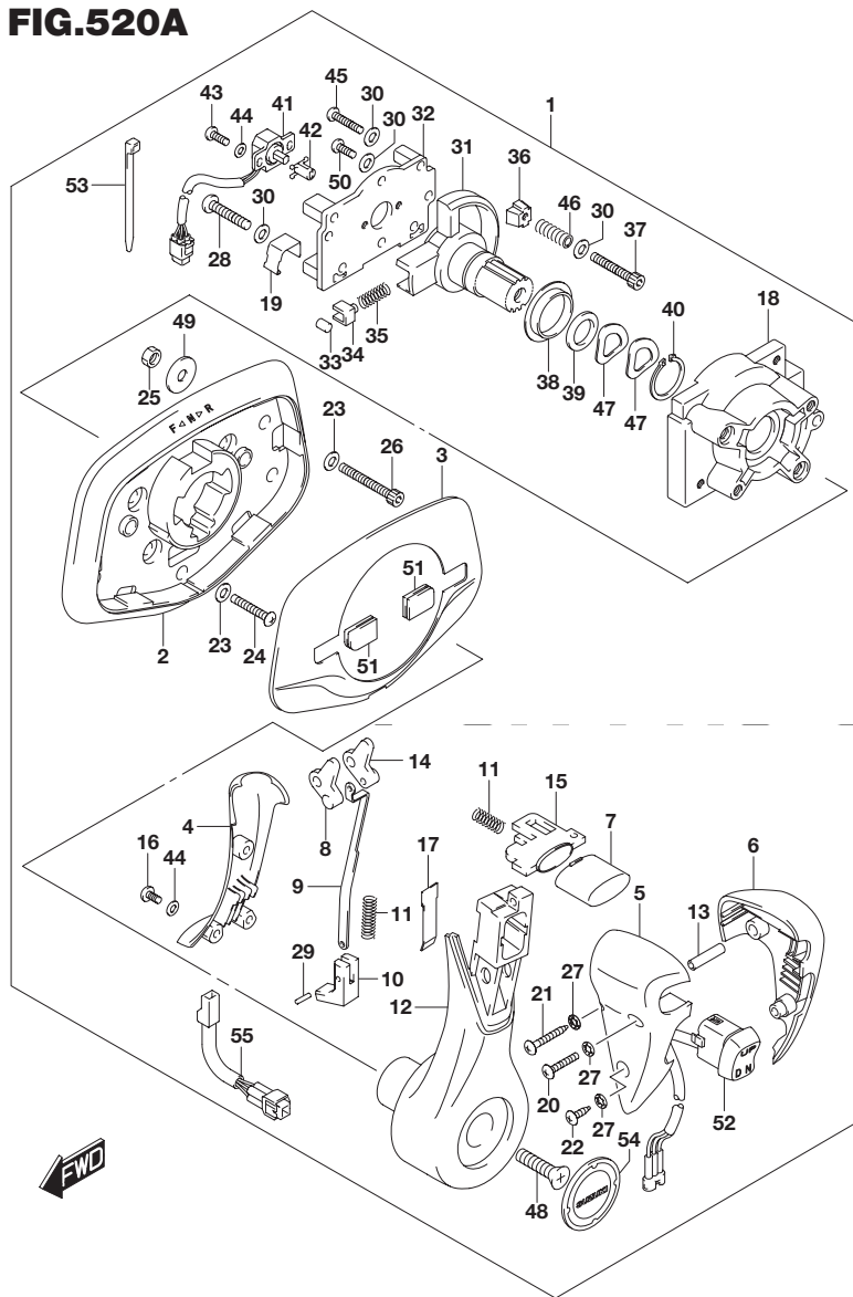
FIG.520A (1-F-6) オプション:フラッシュ マウントリモコン
