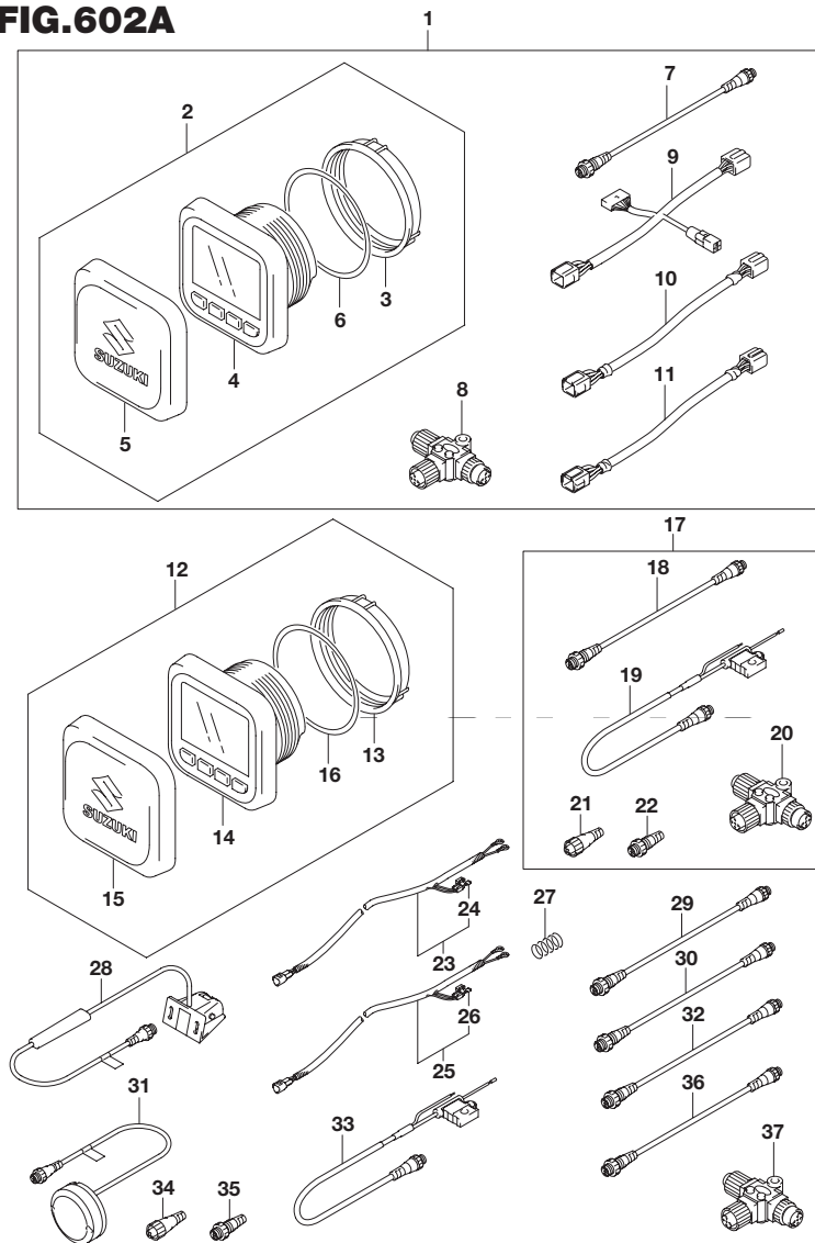
FIG.602A (1-G-8) オプション:マルチ ファンクション ゲージ(2)
