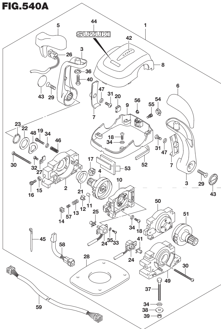
FIG.540A (1-F-13) オプション:リモートコントロール アッシ デュアル
