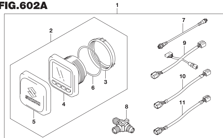
FIG.602A (1-G-9) オプション:マルチ ファンクション ゲージ(2)
