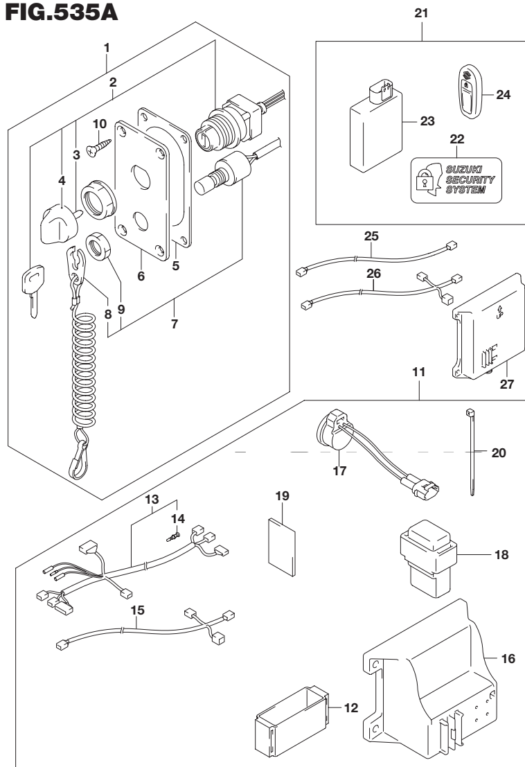
FIG.535A (1-F-12) オプション:キー レス スタート
