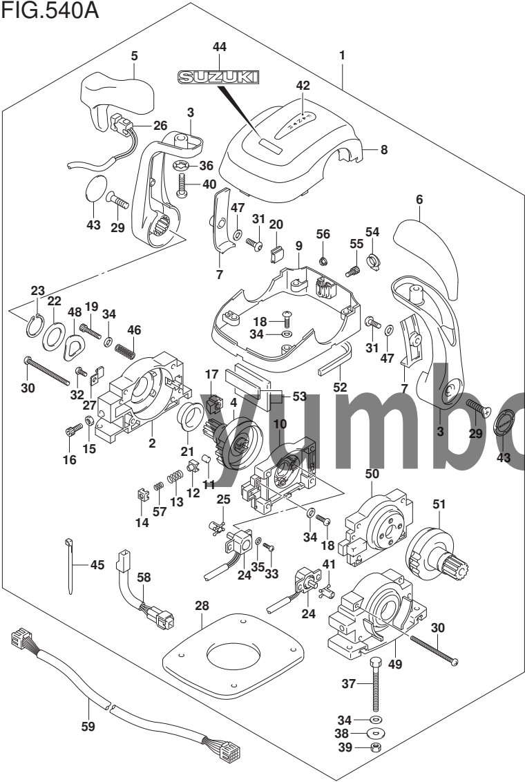
FIG. 540A (1-F-15) オプション:リモート コントロール アツシ デュアル
