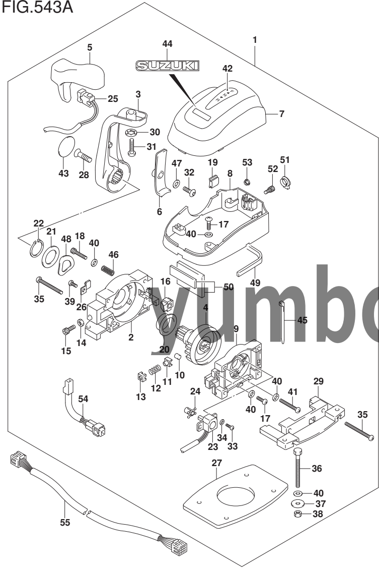
FIG. 543A (1-G-4) オプション:リモート コントロール アツシ シングル
