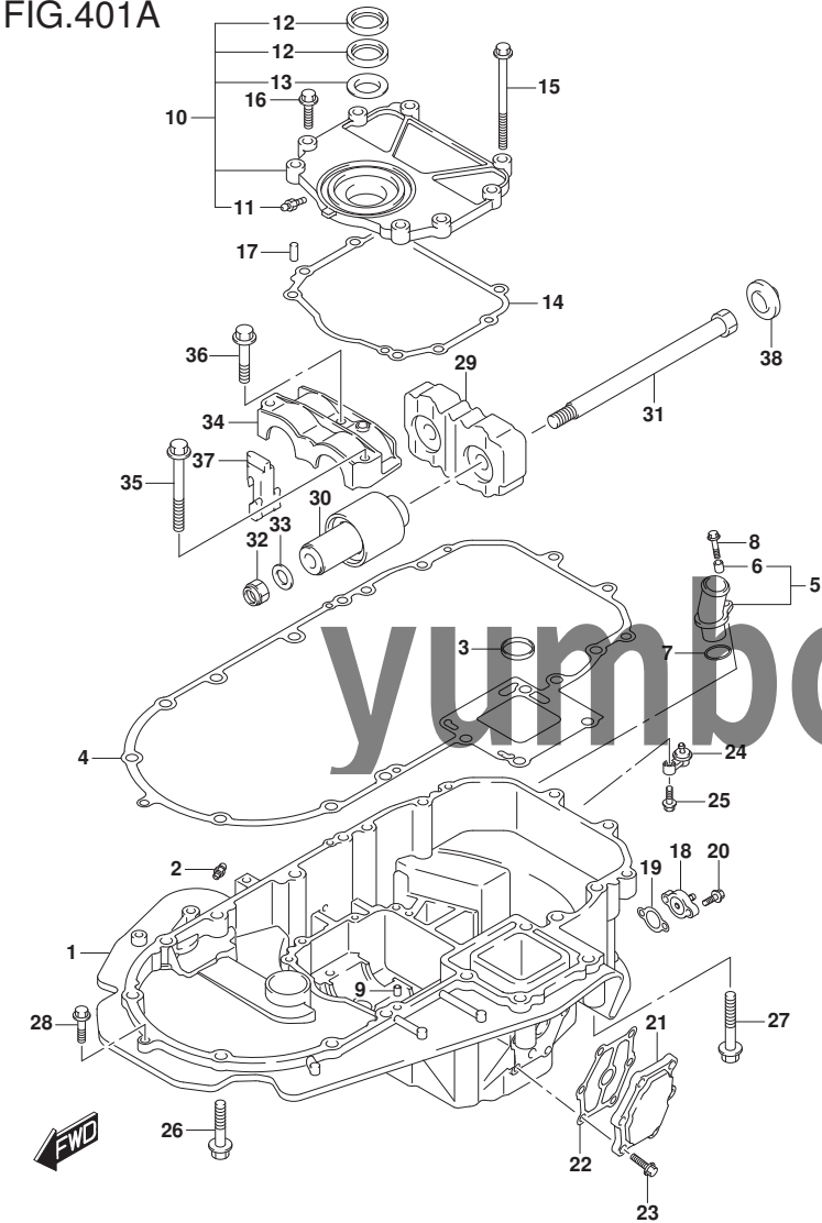
FIG. 401A (1-E-7) エンジンホルダー
