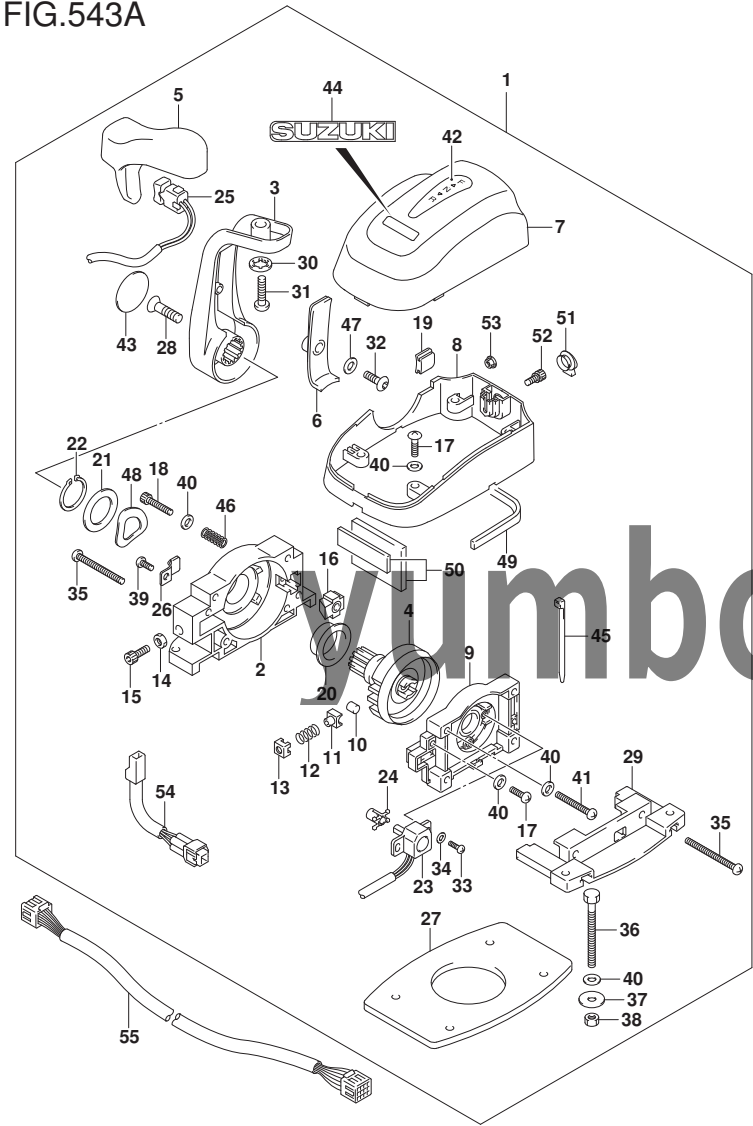
FIG. 543A (1-G-2) オプション:リモート コントロール アツシ シングル
