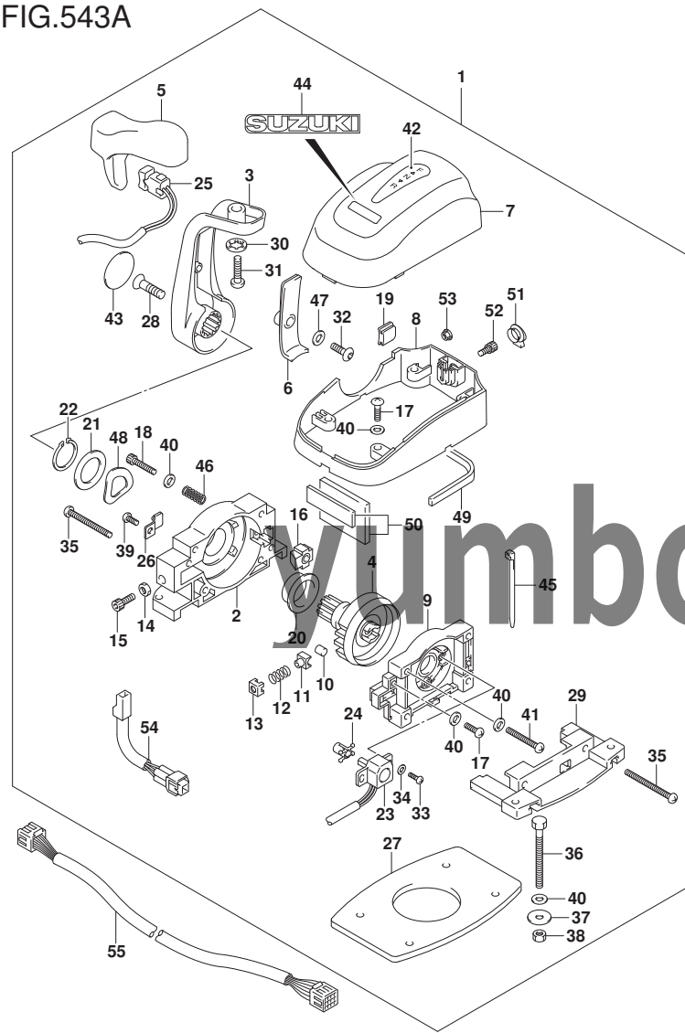
FIG. 543A (1-G-3) オプション:リモート コントロール アッシー シングル
