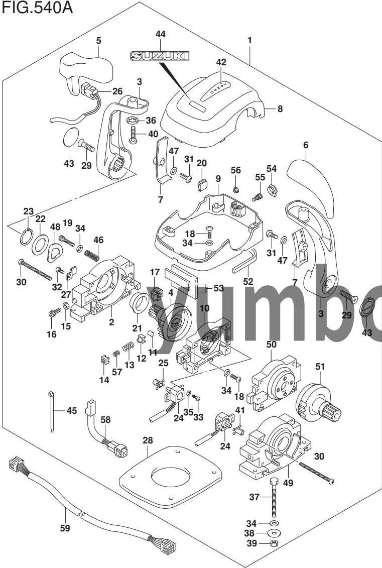
FIG. 540A (1-F-14) オプション:リモート コントロール アツシ デュアル
