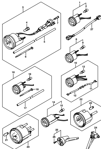
DF200A_000_016_501A OPT METER
