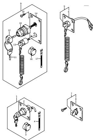
DF25 000_036 OPT-SWITCH-C
