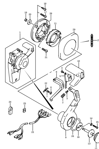
DF25 000_039 OPT-CONCEALED REMOCON (1)-C
