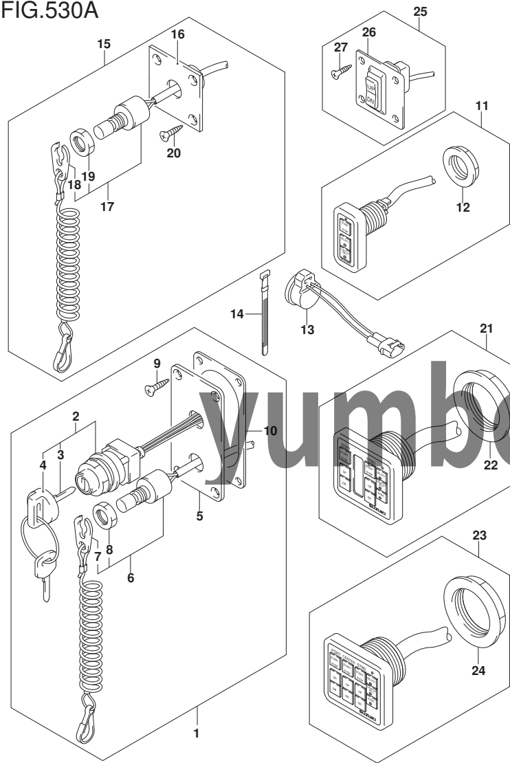
FIG. 530A (1-J-2) オプション:スイッチ
