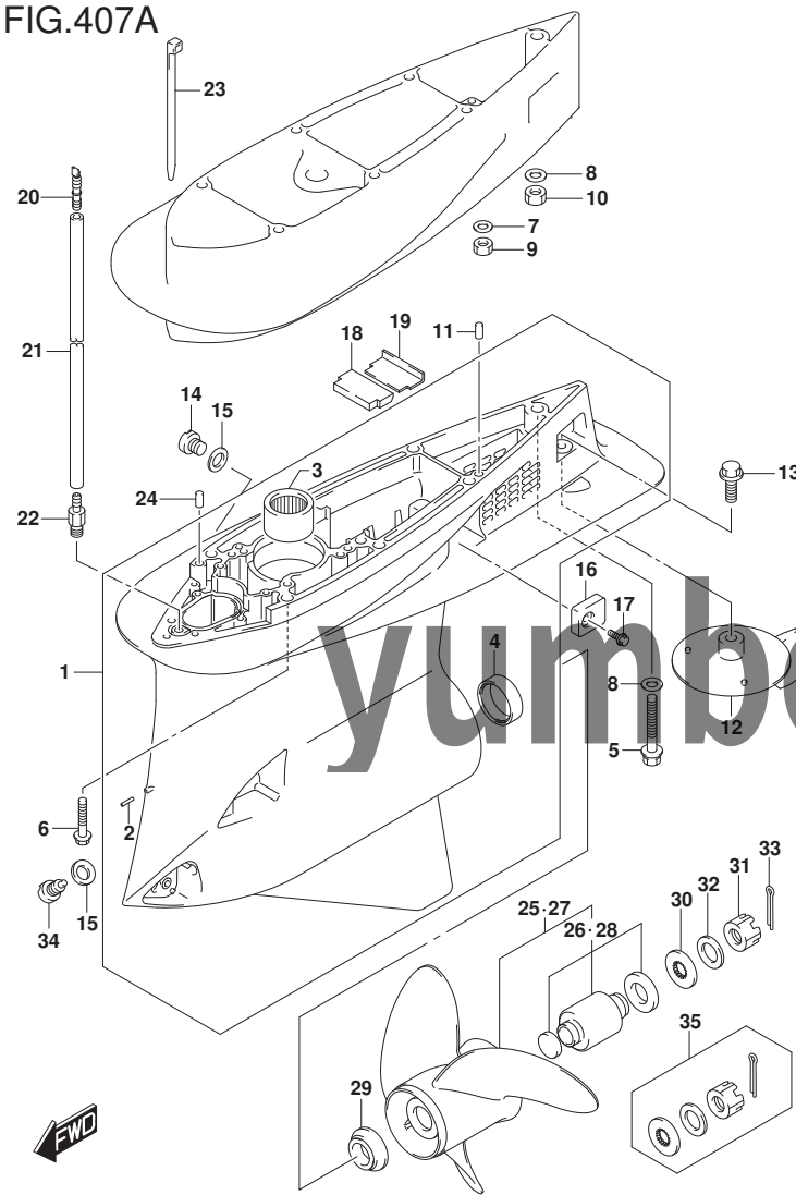
FIG. 407A (1-H-7) ギヤ ケース (DF300A)
