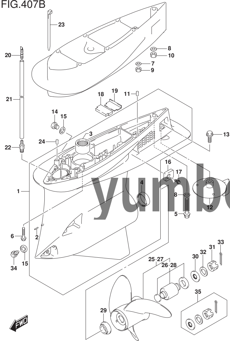
FIG. 407B (1-H-13) ギヤ ケース (DF250A)
