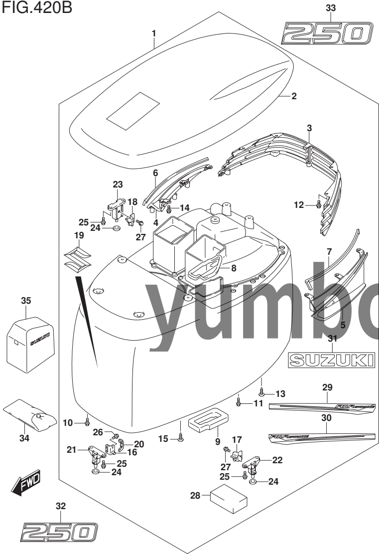
FIG. 420B (1-I-9) エンジン カバー (DF250A)
