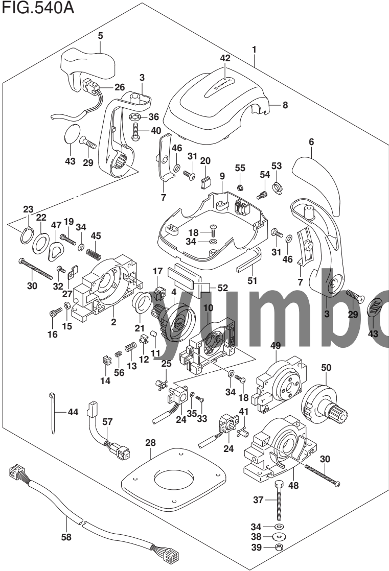
FIG. 540A (1-J-8) オプション:リモート コントロール アツシ デュアル
