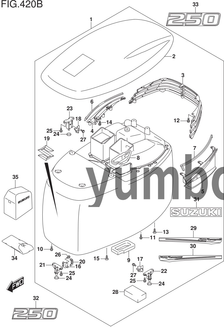
FIG. 420B (1-I-8) エンジン カバー (DF250A)
