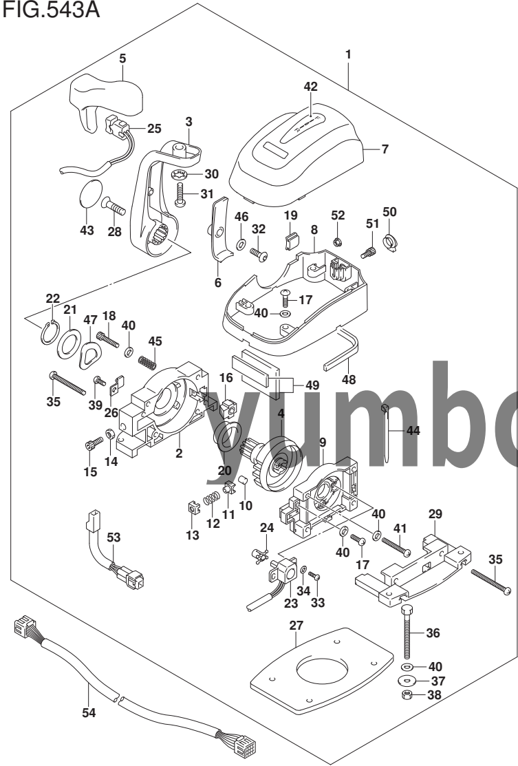
FIG. 543A (1-J-11) オプション:リモート コントロール アッシー シングル
