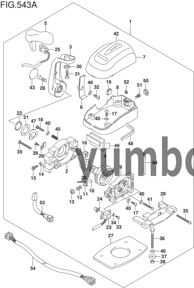
FIG. 543A (1-J-10) オプション:リモート コントロール アツシ シンク
