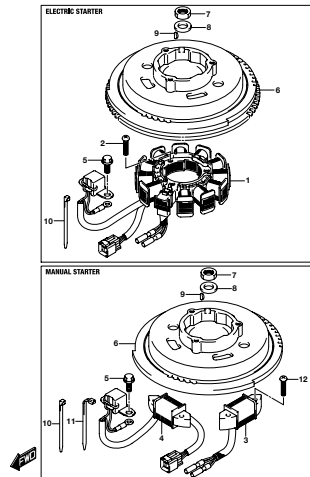
DPF SA_NKD_017_303A MAGNETO
