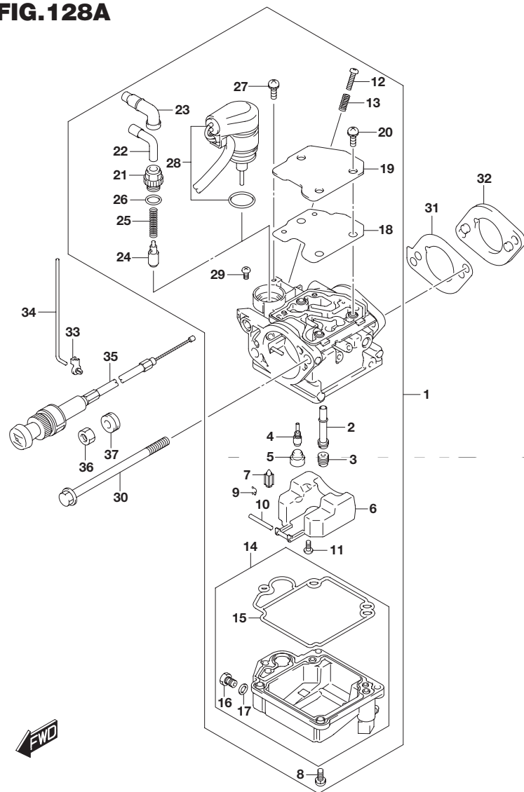
FIG.128A (1-B-8) キャブレタ(DF8A N00)
