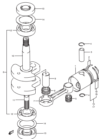
DT2.2 000_002 CRANKSHAFT
