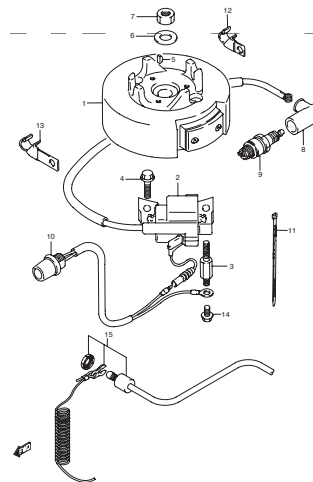
DT2.2 000_007 MAGNETO
