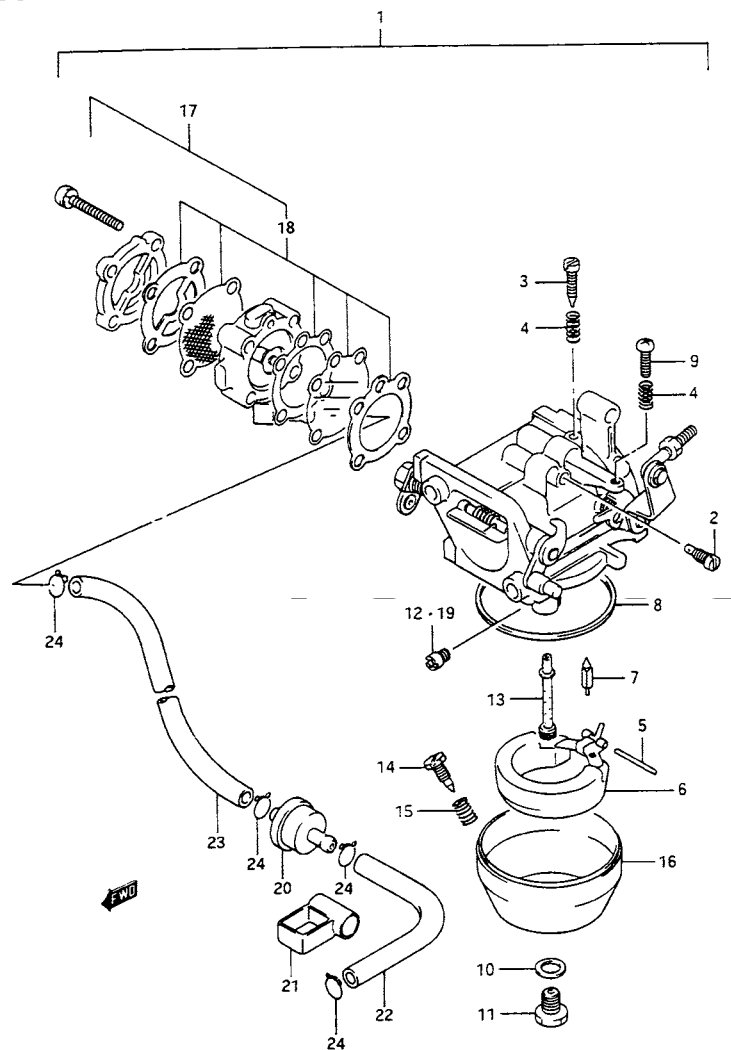
見出番号 品 番 品 名 使用個数 備 考 標準 作業時間 1 13200-92D31 キャブレタアッシ 1 ←13200-92D02 0.8 2 09492-60011 ・ジェット,パイロット,60 1 ←09492-60005 3 13279-90000 ・アジャスタ 1 4 13268-96110 ・スプリング 1 5 13254-98100 ・ピン,フロート 1 6 13250-98110 ・フロート 1 0.9 7 13371-98100 ・ニードル 1 8 13251-98100 ・ガスケット,フロートチャンバ 1 9 13267-93900 ・スクリュ,スロットルストップ 1 10 13343-98100 ・ガスケット 1 11 13613-98100 ・ボルト 1 12 09491-20011 ・ジェット,メイン(102.5) 1 0.9 13 13235-91D00 ・ノズル,メイン 1 ←13235-92D00 14 13616-93900 ・アジャスタ 1 15 13268-96111 ・スプリング 1 ←13268-93520 16 13245-98110 ・フロートチャンバー 1 17 15100-92D11 ・ポンプセット 1 ←15100-92D10 0.9 18 15170-93911 ・ダイヤフラムセット,フューエルポンプ 1 ←15170-93920 0.9 19-1 09491-92005 ジェット,メイン,92.5 1 OPT 19-2 09491-97004 ジェット,メイン(97.5) 1 OPT, ←09491-97007 19-3 09491-21019 ジェット,メイン,107.5 1 OPT 20 15410-98500 フィルタ,フューエル 1 21 15811-92D00 プロテクタ,フューエルホース 1 22 09352-50903-600 ホース,5X9X600 1 (CONN→FILTER) L:600→40 23 09352-50903-600 ホース,5X9X600 1 (FILTER→PUMP) L:600→175 24 09401-08410 クリップ 4
