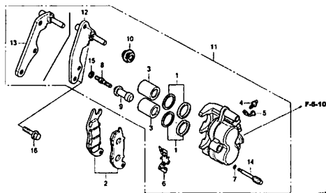
リヤーブレーキキャリパー
