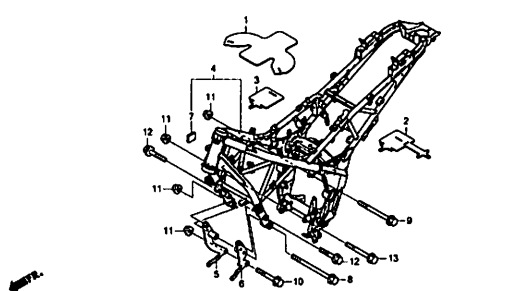
フレームボディ
