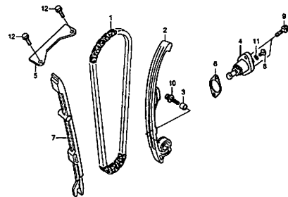
カムチェーン/テンショナー
