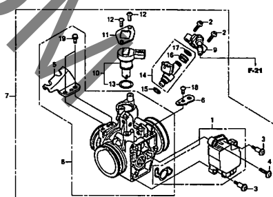
スロットルボディ
