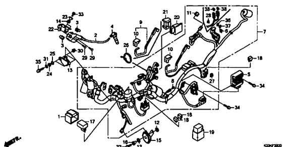
ワイヤーハーネス
