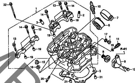
シリンダーヘッド
