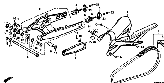
スウィングアーム
