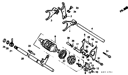
E-15 ギヤースhiftドラム E8
