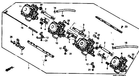
E-16 キャブレター (ASSY.) E10
