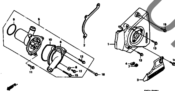
E-12 クランクケース E4
