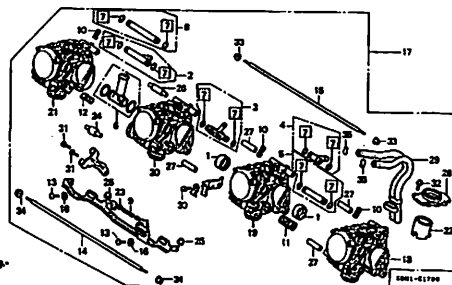
E-17 キャブレター (ASSY.) E14
