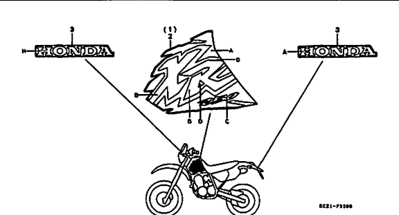
F-32 マーク (XR250S) J7
