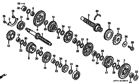
E-13-1 トランスミッション (CBR250RJ・RK) G3
