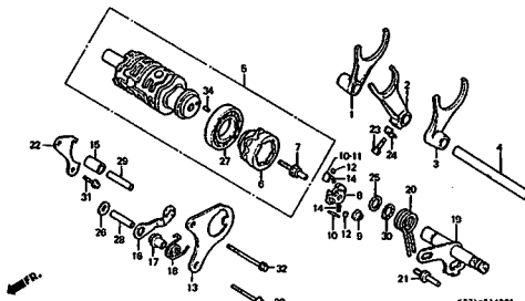
E-14 ギヤシフトドラム G5
