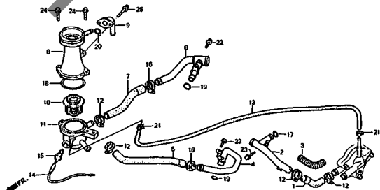
E-15 ウォーターパイプ・サーモスタット (CBR250FG・FG-YA・RH) G8
