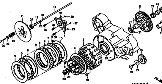
E-5-1 クラッチ (2) E11
