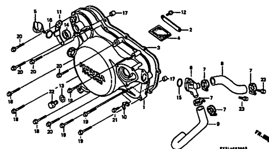
E-5 クラッチ (1) E9
