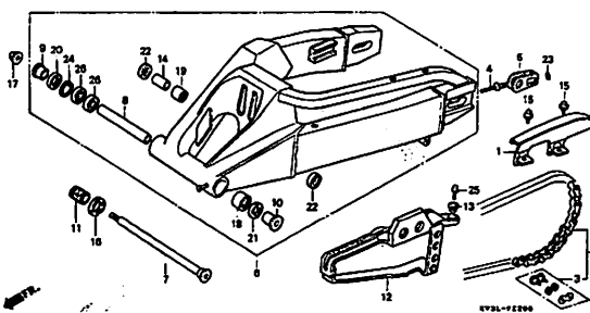
F-22 スウィングアーム・チェーンケース J1
