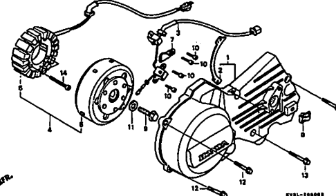
E-6 L. クランクケースカバー・ A.C. ジェネレーター E13
