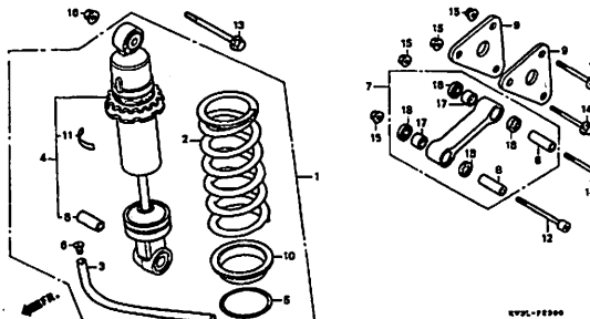
F-23 リヤクッション (1) J3
