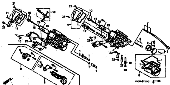
E-13-1 キャブレター (構成部品) F8
