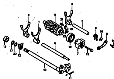
E-11 ギヤースhiftドラム・ギヤースhiftフォーク F3
