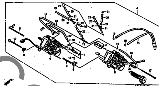
E-13 キャブレター (ASSY.) F6
