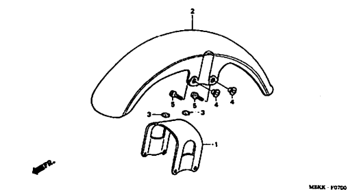
フロントフェンダー
