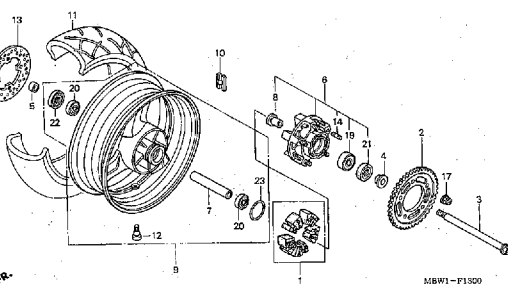
リヤーホイール(1)
