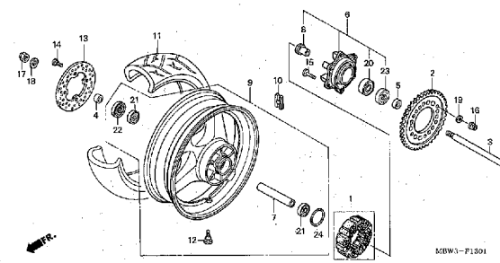
リヤーホイール(2)
