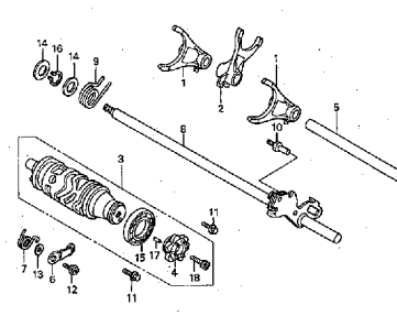
ギヤーシフトドラム
