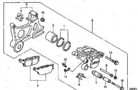
リヤーブレーキキャリパー
