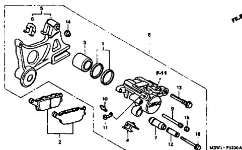
リヤブレーキキャリパー
