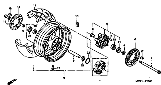
リヤホイール (CBR600FX/Y)
