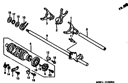
ギヤーシフトドラム/ギヤーシフトフォーク
