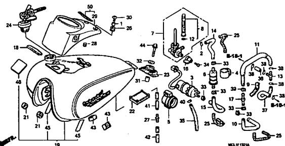
フューエルタンク/フューエルポンプ (DC4-DC8)
