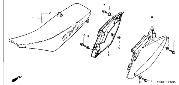
シート/サイドカバー (CRF450R2, 3, 4)
