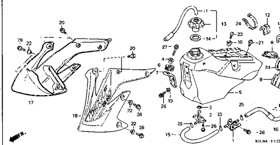
フューエルタンク (CRF450R5, 6, 7, 8)
