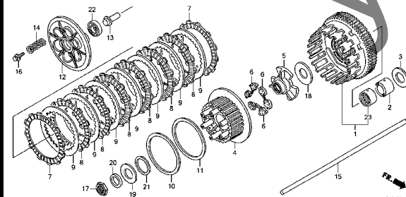
クラッチ (CB1300A/ADE, F, G)
