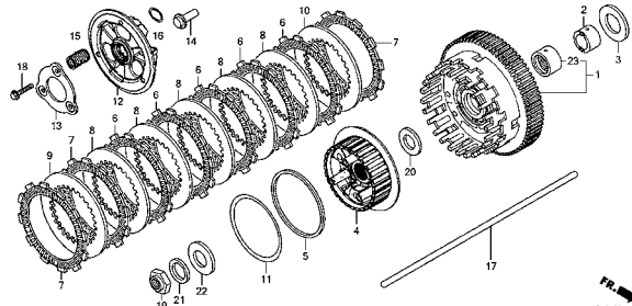
クラッチ (CB1300ADJ, K/SPK)
