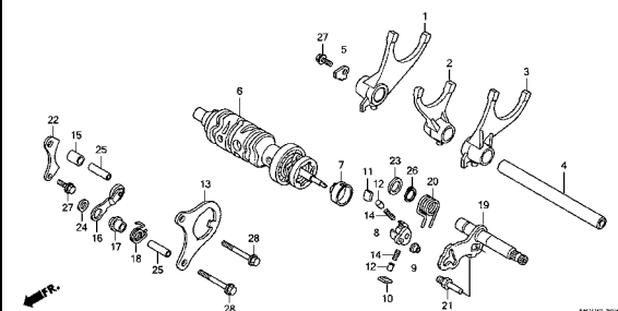
ギヤーシフトドラム/ギヤーシフトフォーク
