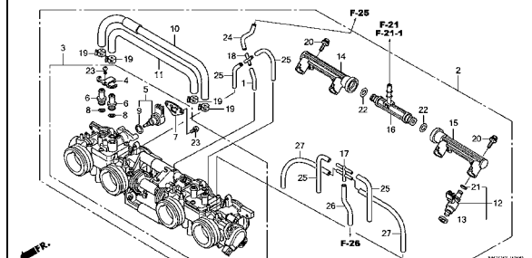
スロットルボディ
