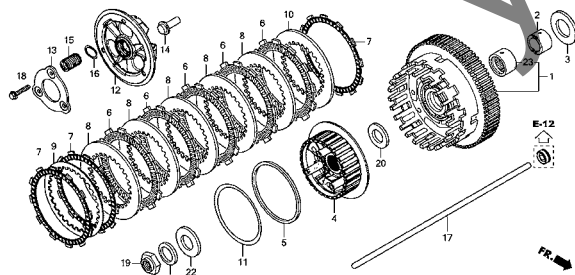
クラッチ
