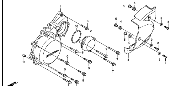
L. クランクケースカバー
