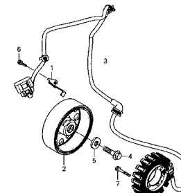
ジェネレーター
