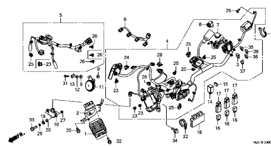
ワイヤーハーネス
