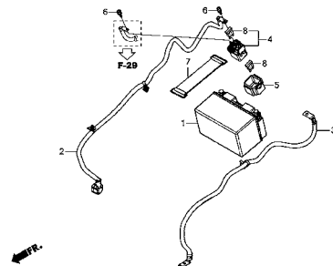
バッテリー
