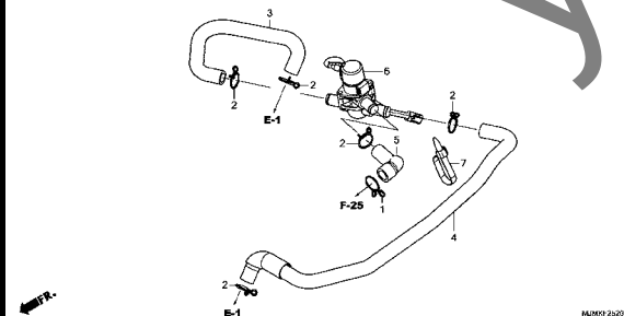
エアーインジェクションコントロールバルブ
