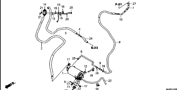
キャニスター
