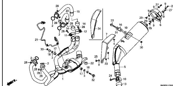
エキゾーストマフラー
