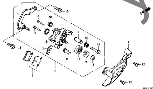
パーキングブレーキキャリパー
