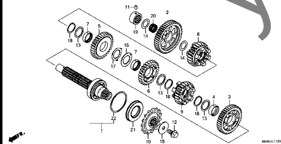
ミッション(カウンターシャフト)
