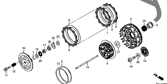
クラッチ
