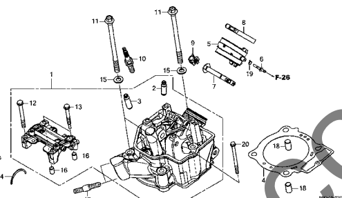
シリンドー
