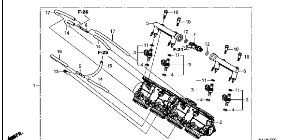
スロットルボディ
