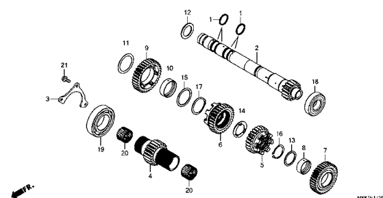
トランスミッション(メインシャフト) (CRF1000D/D2/DL2)
