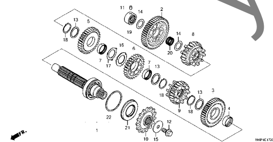
ミッション(カウンターシャフト)
