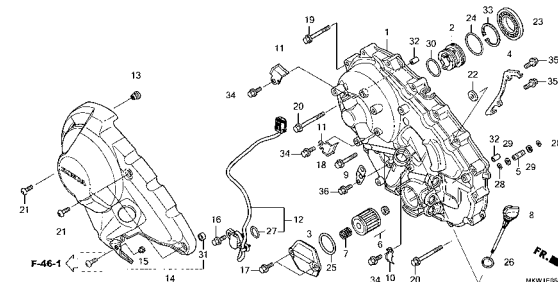
リニアソレノイド
