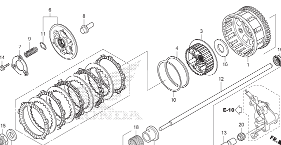
E-8-1 CLUTCH(CBR250S3A)
