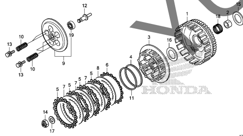
CLUTCH
