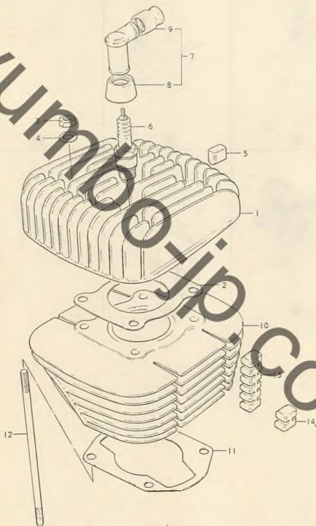
FIG. 1 シリンダ
