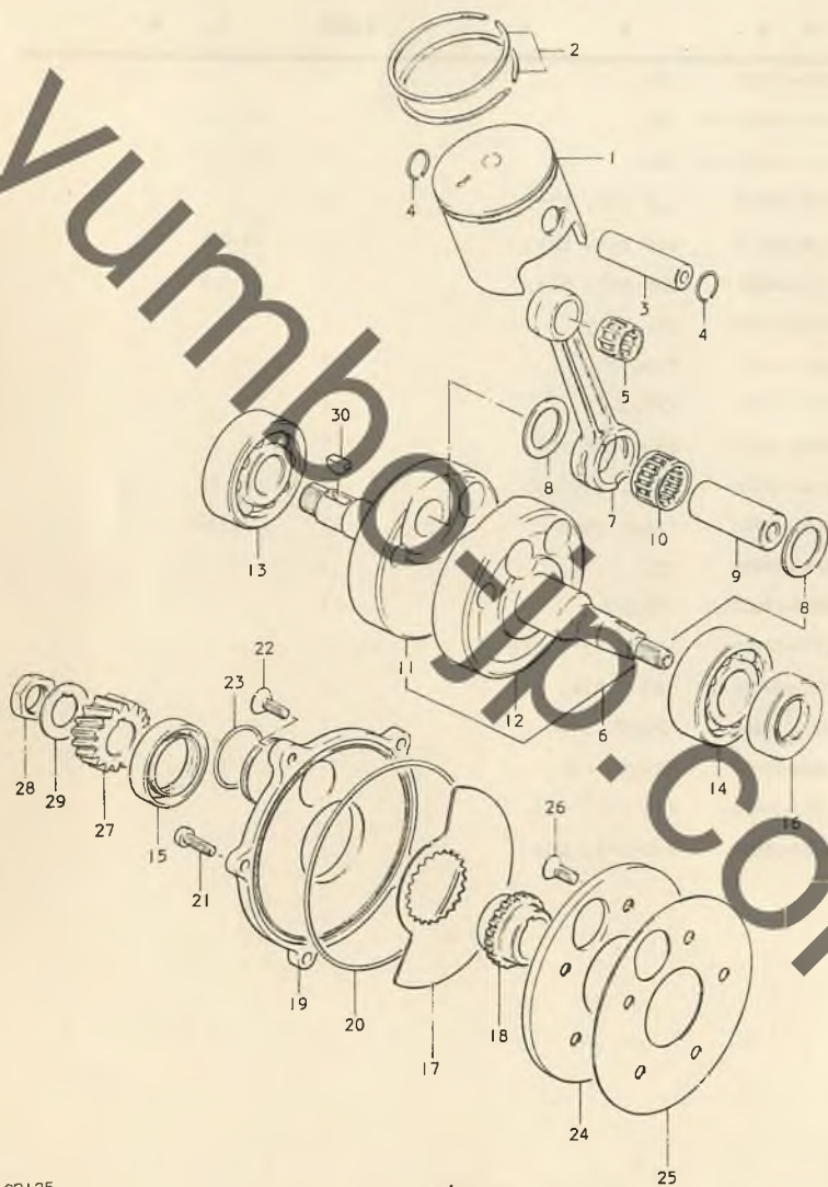
FIG. 4 クランクシャフト
