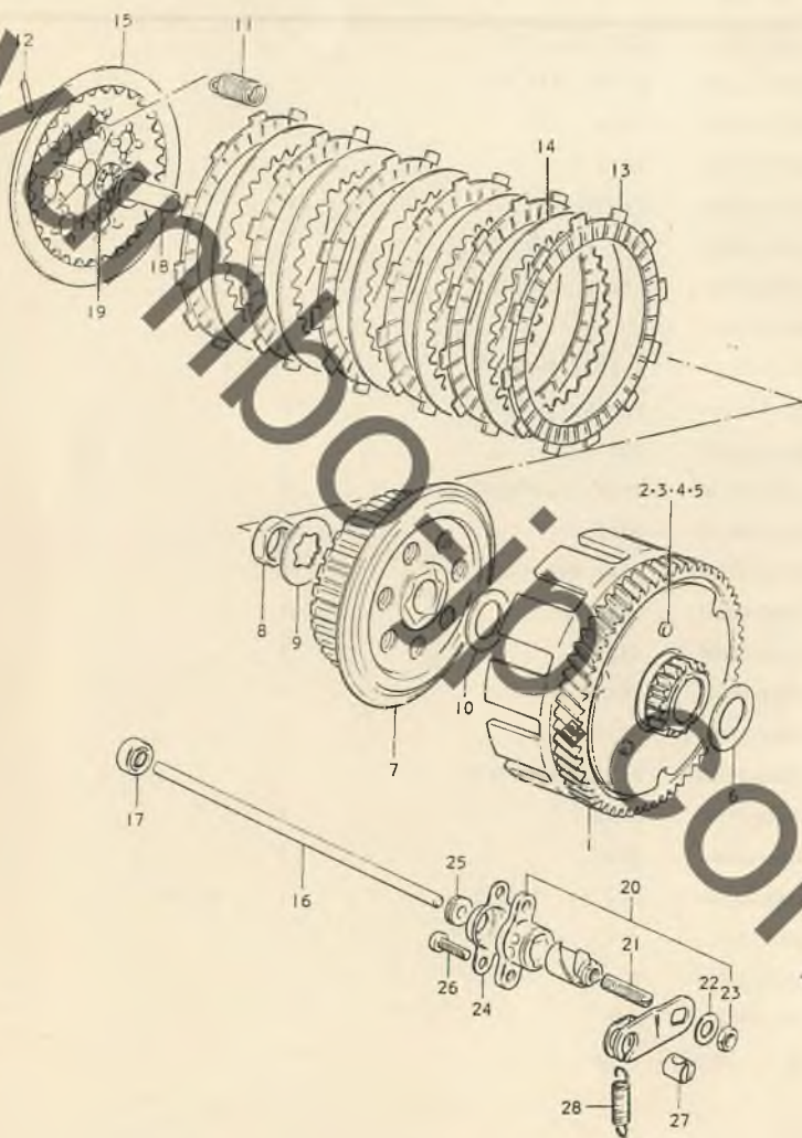
FIG. 9 クラッチ
