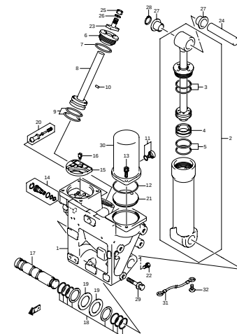
DF200 225 250 000_035 TRIM CYLINDER-C
