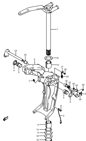
DF200 225 250 000_033 SWIVEL BRACKET-C
