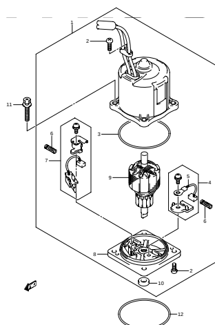
DF200 225 250 000_037 PTT MOTOR-C
