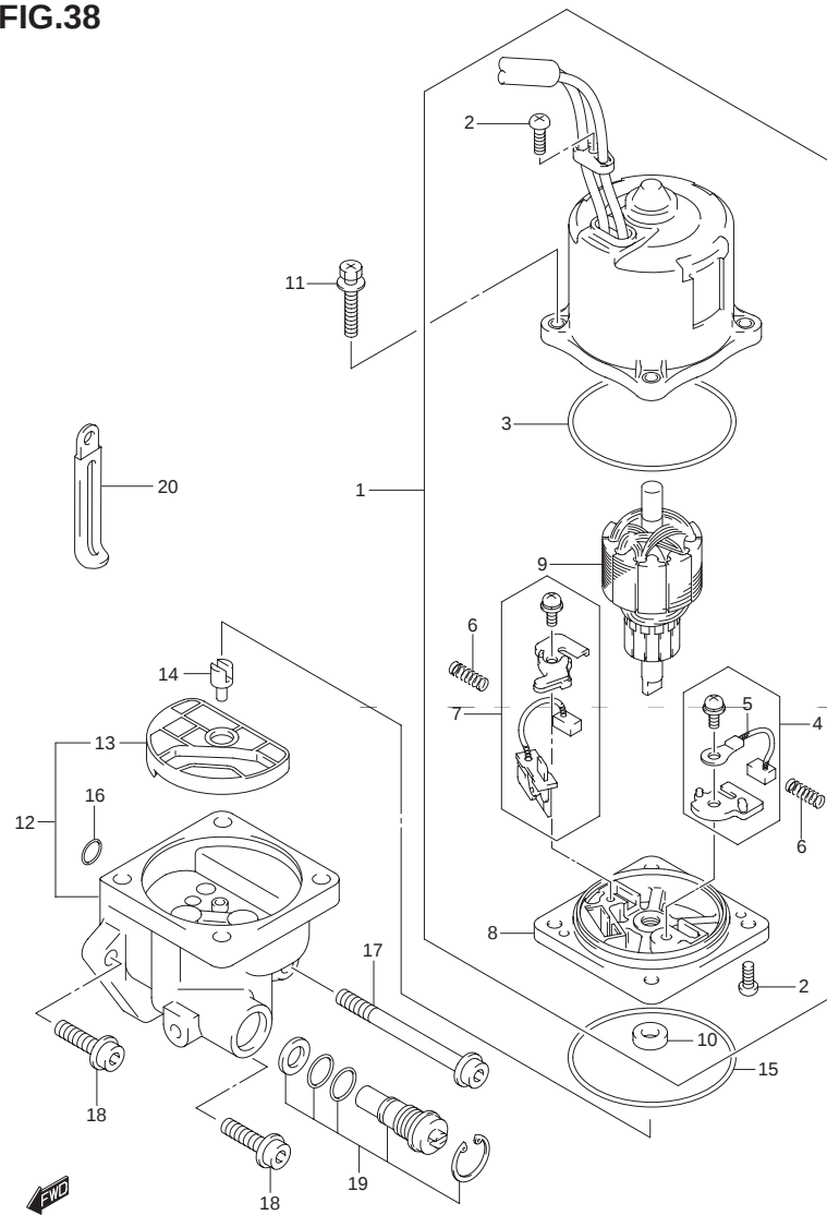
FIG.38 (H-15) PTT モータ (DF200TL)
