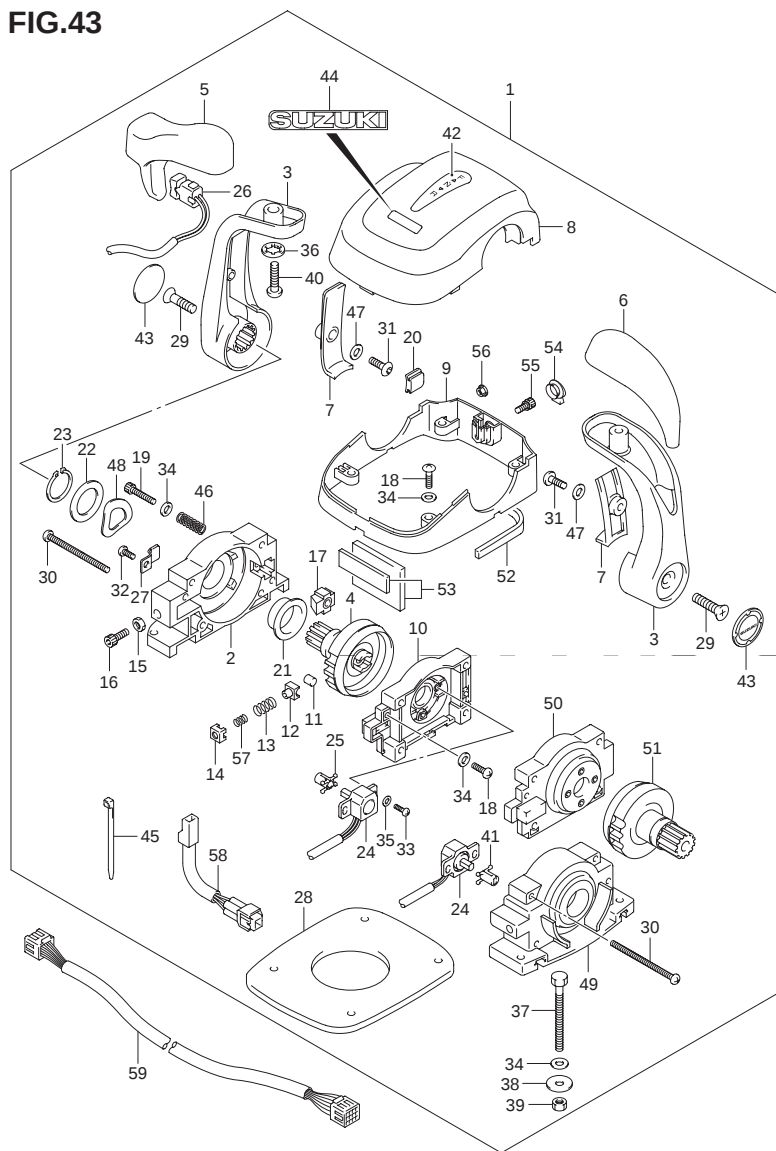
FIG.43 (1-H-2) オプション:リモートコントロール アッシ デュアル
