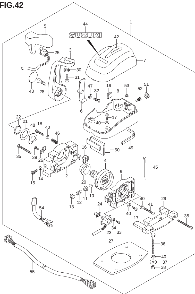
FIG.42 (1-G-13) オプション:リモートコントロールアッシ シングル
