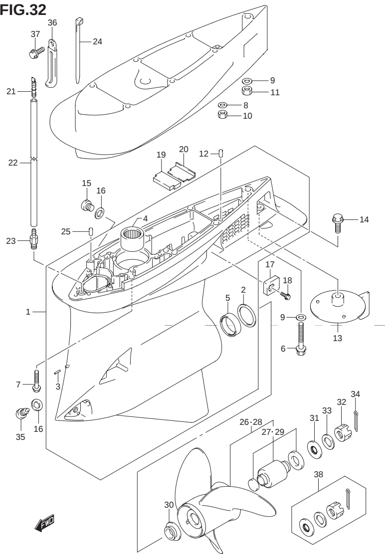
FIG.32 (1-F-6) ギヤ ケース
