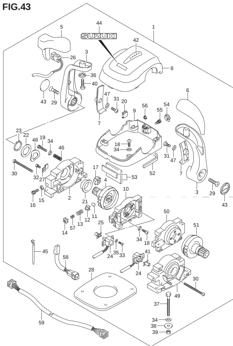
FIG.43 (1-H-3) オプション:リモートコントロール アッシ デュアル
