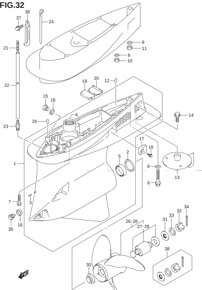
FIG.32 (1-F-5) ギヤ ケース
