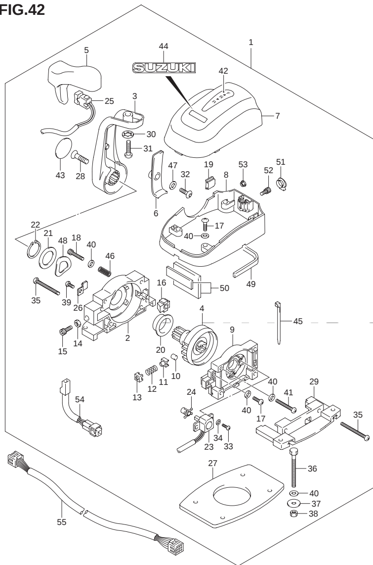
FIG.42 (1-G-15) オプション:リモートコントロールアッシ シングル
