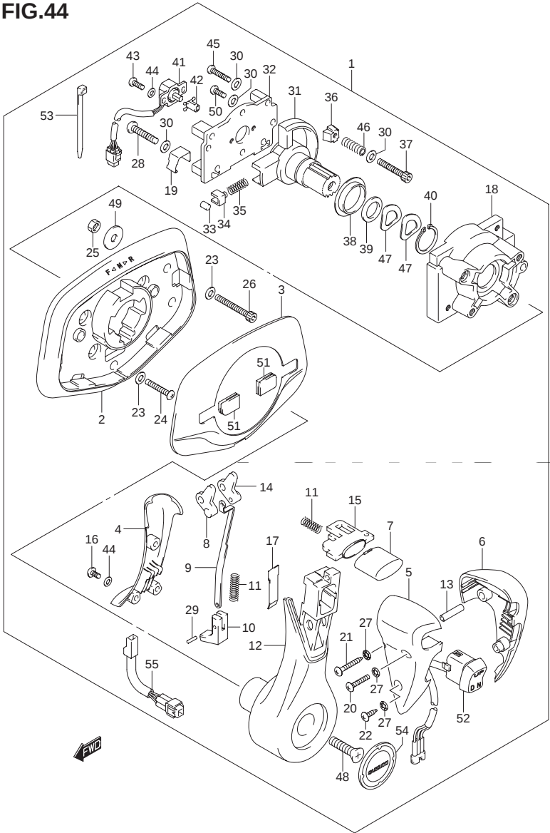
FIG.44 (1-H-7) オプション:フラッシュマウントリモコン
