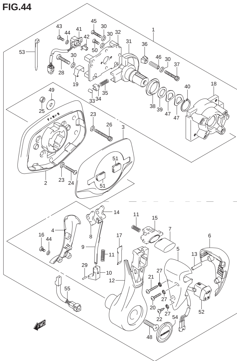
FIG.44 (1-H-5) オプション:フラッシュマウントリモコン
