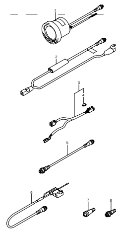
DF300A_000_014_037 METER
