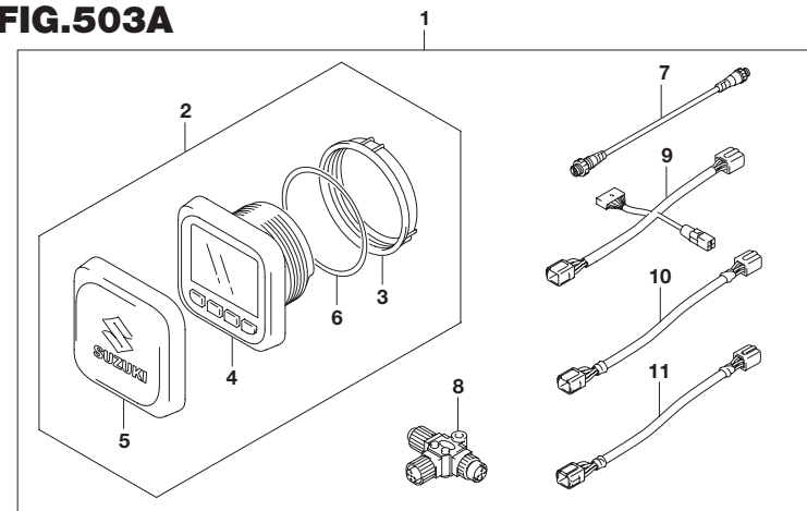
FIG.503A (1-I-8) オプション:メータ(2)
