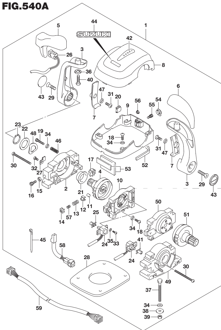
FIG.540A (1-J-6) オプション:リモートコントロールアッシデュアル
