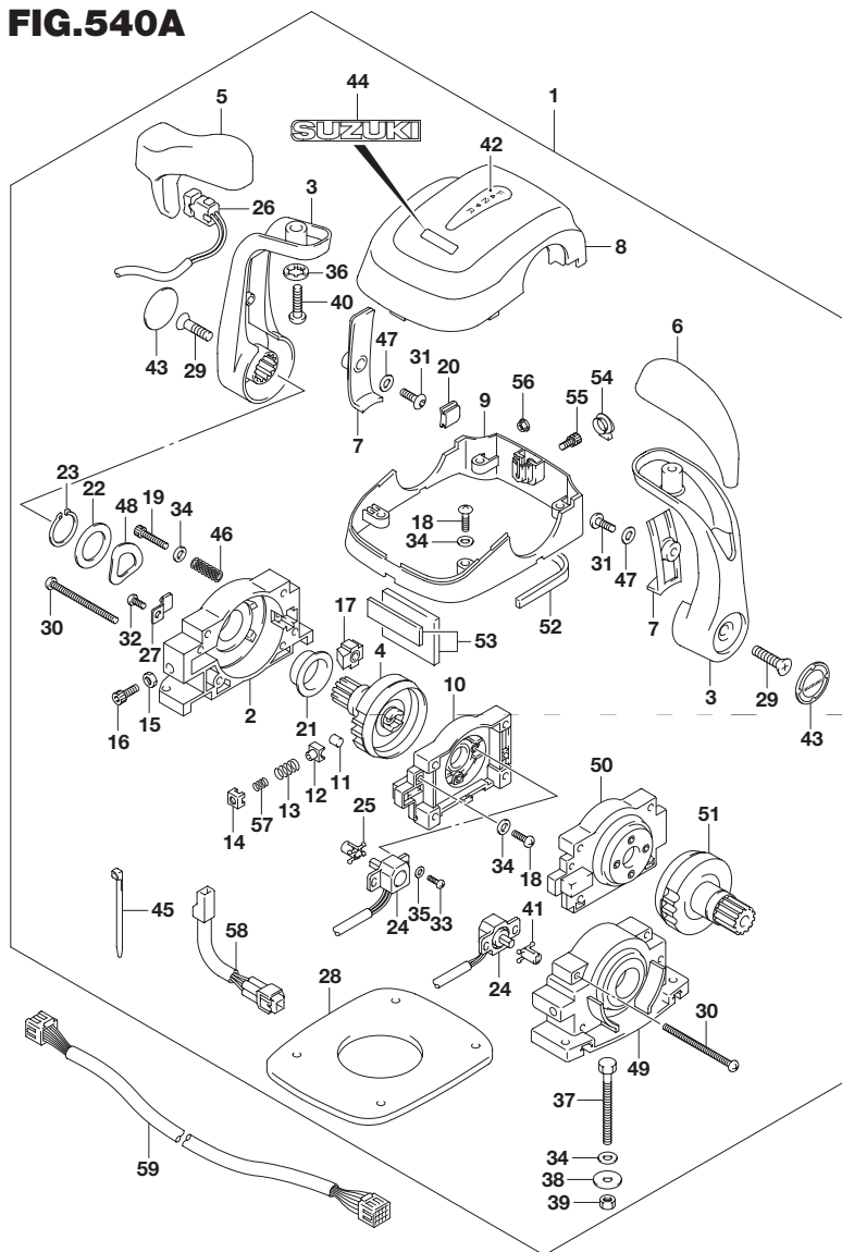
FIG.540A (1-J-5) オプション:リモートコントロールアッシ デュアル
