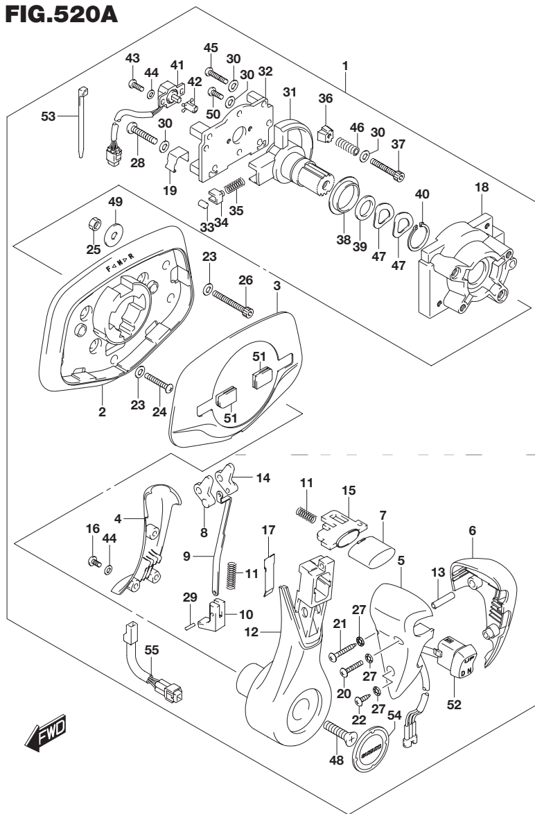
FIG.520A (1-I-11) オプション:フラッシュ マウント リモコン
