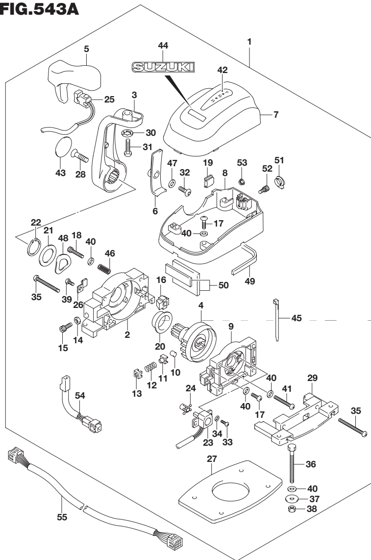
FIG.543A (1-J-8) オプション:リモートコントロール アッシ シングル
