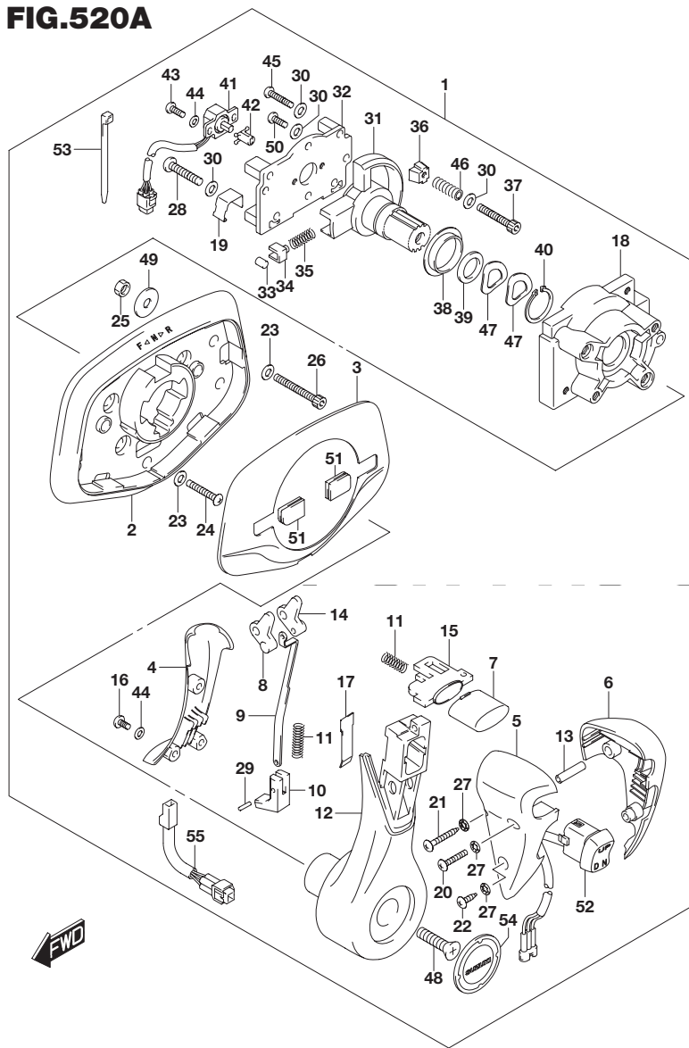
FIG.520A (1-I-10) オプション:フラッシュ マウント リモコン
