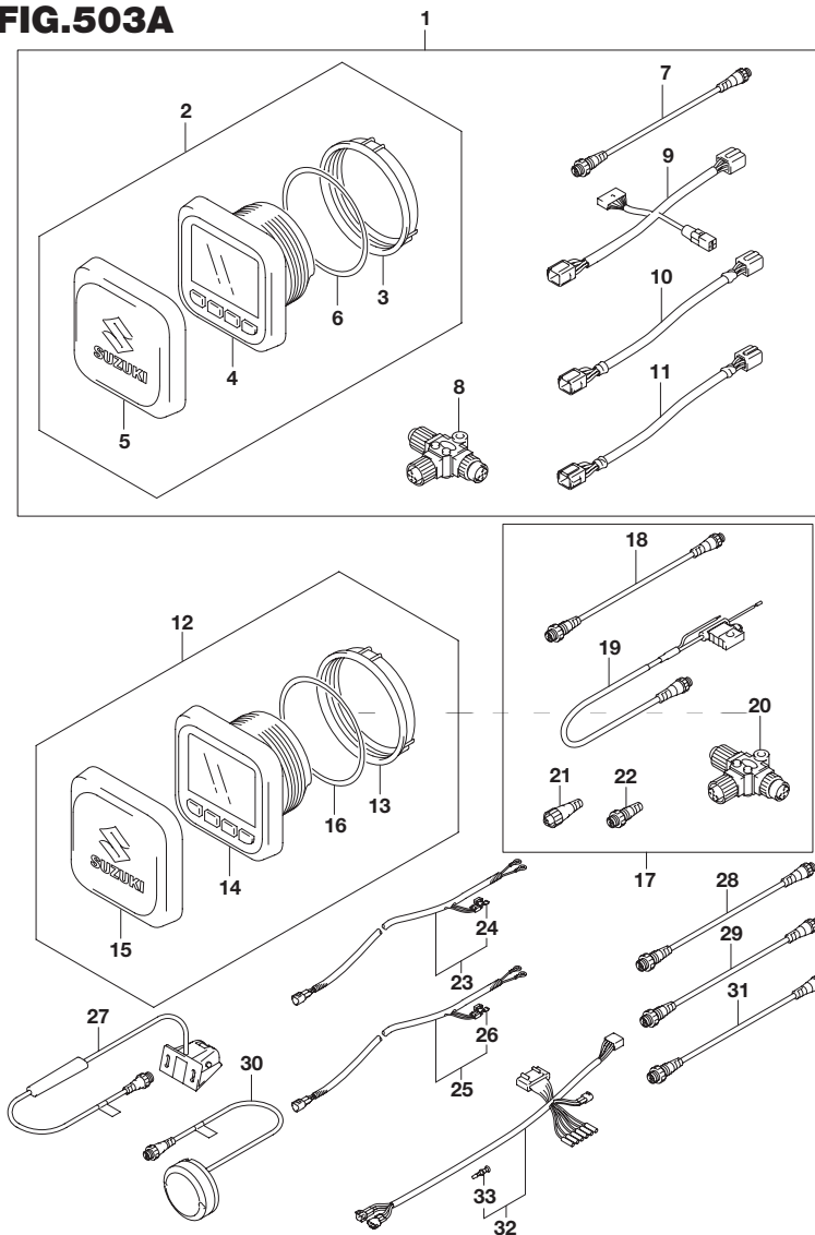
FIG.503A (1-I-7) オプション:メータ(2)
