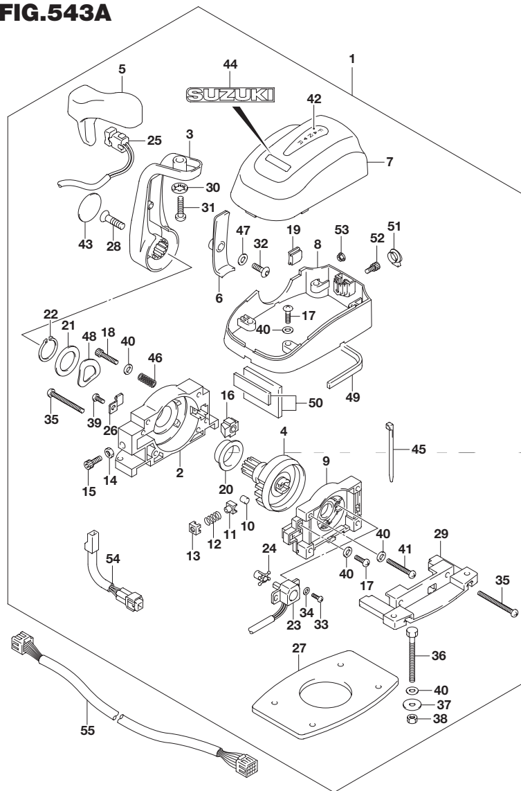
FIG.543A (1-J-10) オプション:リモートコントロールアッシ シングル
