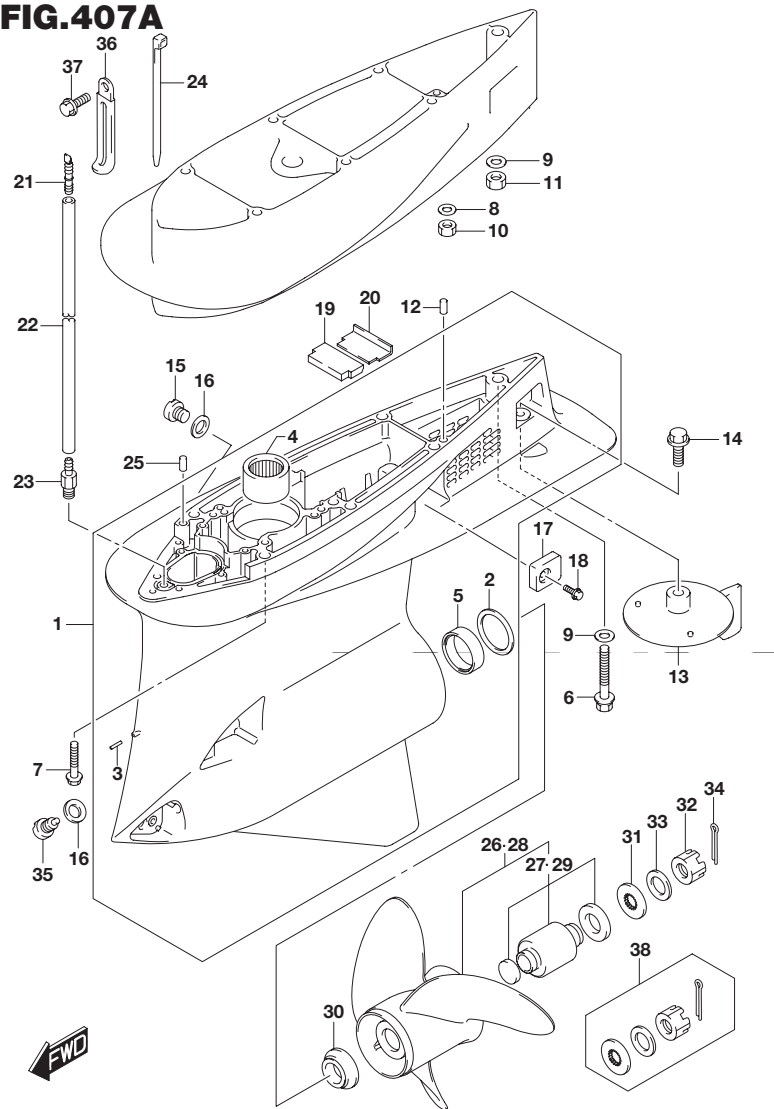
FIG.407A (1-G-9) ギヤ ケース(DF300A:612132マデ ,DF250A:610591マデ)
