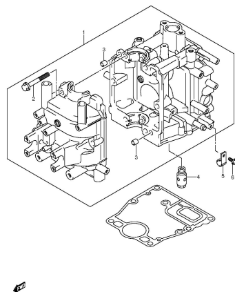
DF8A 9 SA P03 012_002 CYLINDER BLOCK
