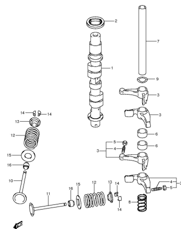
DF8A 9 9A P03 012_009 CAMSHAFT
