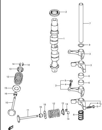
DF8A 9 9A P03 012_011 CAMSHAFT
