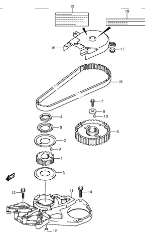
DF8A 9 SA P03 012_007 TIMING BELT
