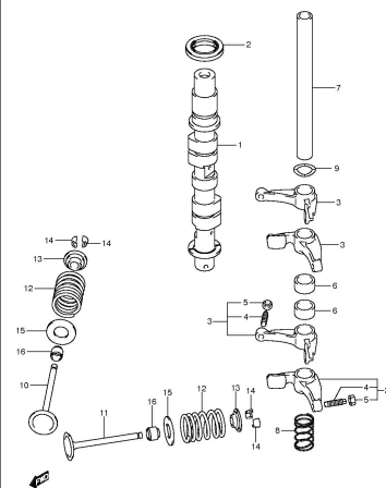
DF8A 9 9A P03 012_010 CAMSHAFT
