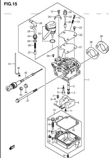
DF8A 9 9A P03 012_015 CARBURETOR
