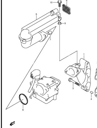
DF8A 9 9A P03 012_012 INLET MANIFOLD
