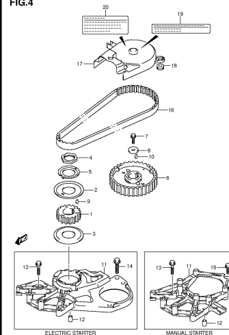
DF8A 9 SA P03 012_004 TIMING BELT
