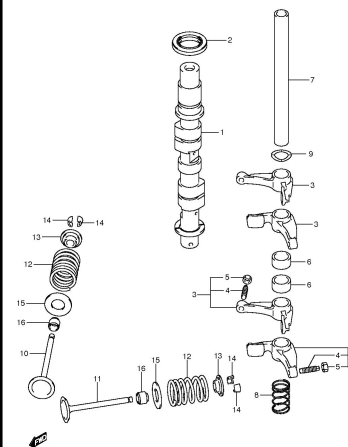
DF8A 9 SA P03 012_008 CAMSHAFT
