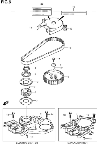
DF8A 9 SA P03 012_006 TIMING BELT
