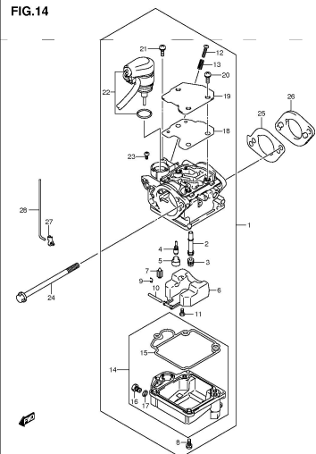
DF8A 9 9A P03 012_014 CARBURETOR
