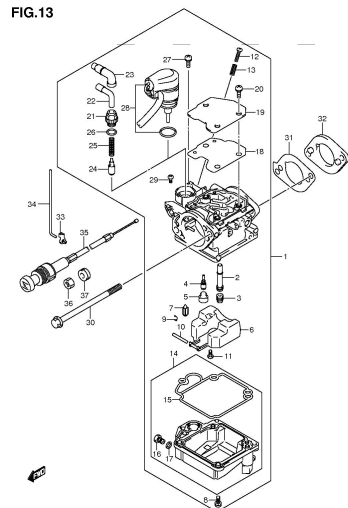
DF8A 9 9A P03 012_013 CARBURETOR
