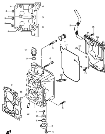
DF8A 9 SA P03 012_001 CYLINDER HEAD
