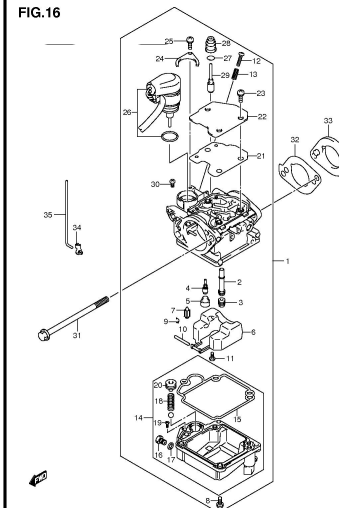
DF8A 9 9A P03 012_016 CARBURETOR
