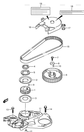
DF8A 9 SA P03 012_005 TIMING BELT
