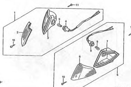
F-18 フロントウinker (SE50MF,MSG,MG・ SE55MSG) J15
