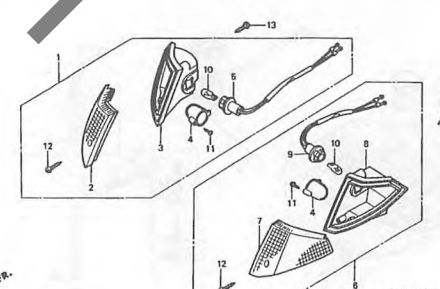
F-18-1 フロントウinker (SE50MSH,MSJ) J16
