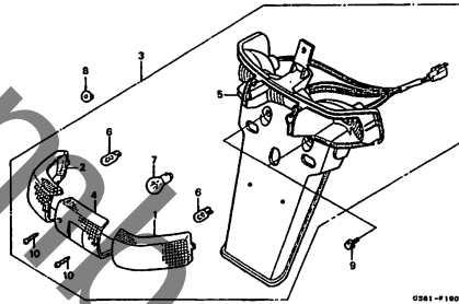
F-21 フレームボディ・リヤフェンダー
