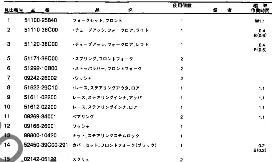
FIG.37 (J-2) フロント フォーク (AJ50P/R/-S)
